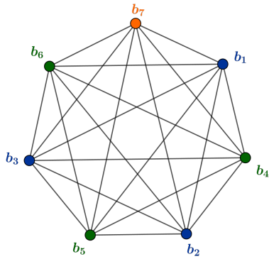
Slika 1.3: SRG(7, 6, 5, 9)
