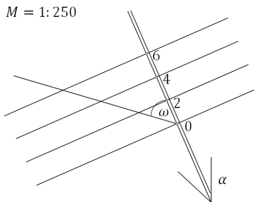
Slika 34: Kotirana projekcija priklopnog kuta
