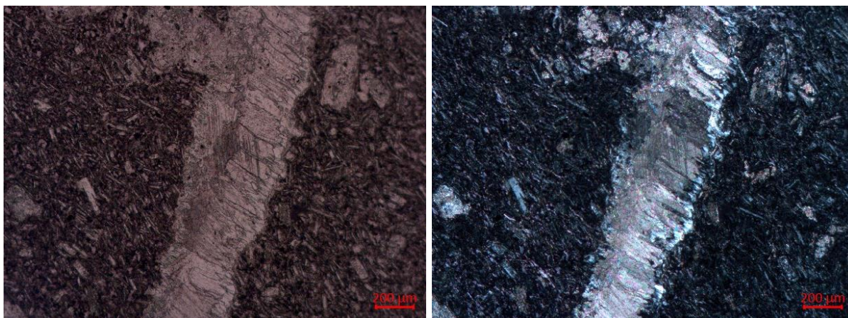
Slika 7.14: Mikrofotografije pukotine uzorka u4 . Lijevo (N-), desno (N+). Kalcitom ispunjena pukotina s kvarcnim rubom. Crvena linija označava 200 \mu\text{m} .
