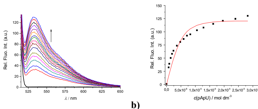
Slika D13. a) Promjene u fluorescencijskom spektru spoja 3a ( c = 5 \times 10^{-7} \text{ mol dm}^{-3} ) tijekom titracije s p\text{ApU} , uz pobudu pri \lambda_{\text{eks}} = 510 \text{ nm} u puferu natrijeva kakodilata ( \text{pH} = 7,0 ; I = 0,05 \text{ mol dm}^{-3} ) pri 25 \text{ }^\circ\text{C}
