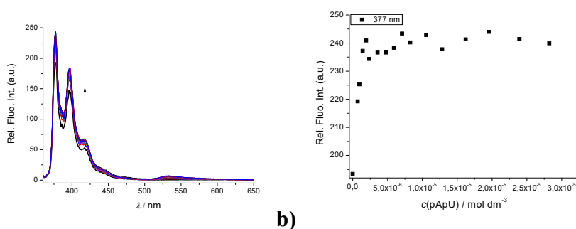
Slika D12. a) Promjene u fluorescencijskom spektru spoja 3a ( c = 5 \times 10^{-7} \text{ mol dm}^{-3} ) tijekom titracije s \text{pApU} , uz pobudu pri \lambda_{\text{eks}} = 348 \text{ nm} u puferu natrijeva kakodilata ( \text{pH} = 7,0 ; I = 0,05 \text{ mol dm}^{-3} ) pri 25 \text{ }^\circ\text{C} ; b) Ovisnost relativnog fluorescencijskog inteziteta spoja 3a o koncentraciji \text{pApU} uz emisiju pri \lambda_{\text{em}} = 377 \text{ nm} u puferu natrijeva kakodilata ( \text{pH} = 7,0 ; I = 0,05 \text{ mol dm}^{-3} ) pri 25 \text{ }^\circ\text{C}
