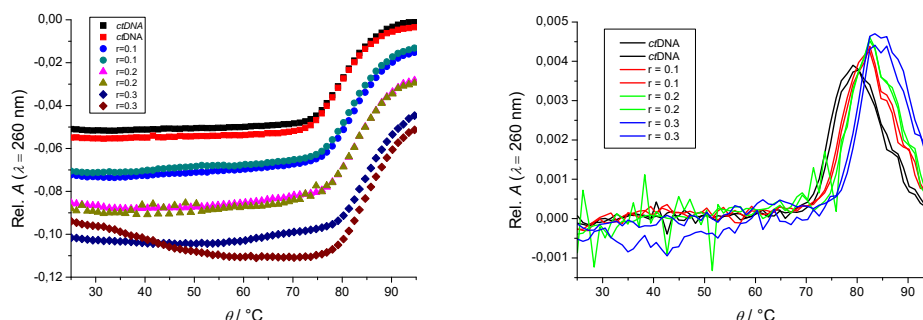
Slika D22. a) Krivulja mekšanja ctDNA ( c=2 \times 10^{-5} mol dm^{-3} ) nakon dodatka spoja 1 pri različitim omjerima r = [\text{spoj}]/[\text{polinukleotid}] u puferu natrijeva kakodilata ( pH=7,0; I=0,05 mol dm^{-3} ); b) Maksimumi prvih derivacija krivulja mekšanja ctDNA ( c=2 \times 10^{-5} mol dm^{-3} ) nakon dodatka spoja 1 pri različitim omjerima r = [\text{spoj}]/[\text{polinukleotid}] u puferu natrijeva kakodilata ( pH=7,0; I=0,05 mol dm^{-3} )
