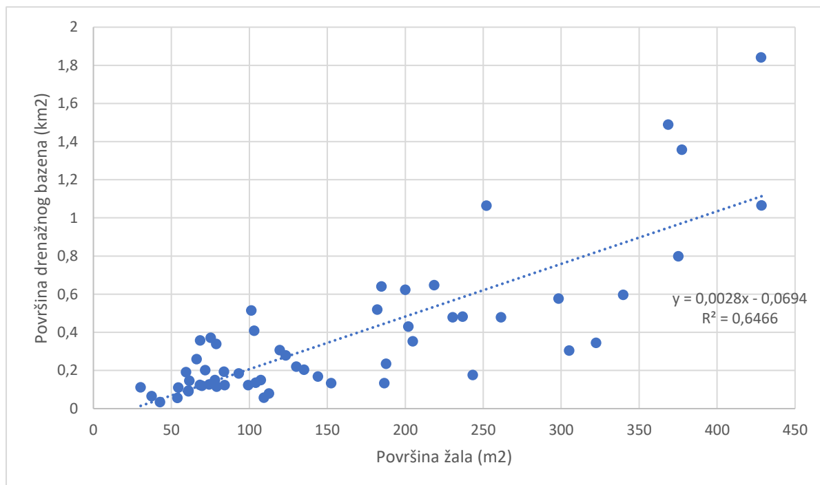
Sl. 27. Korelacija površina žala i površina drenažnih bazena bez antropogenog utjecaja
