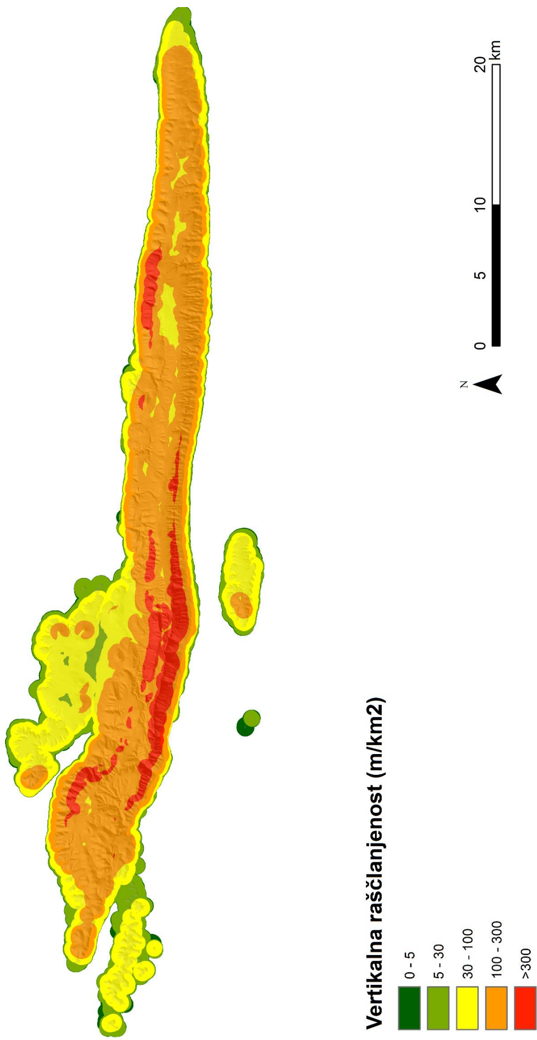
Sl. 7. Karta vertikalne raščlanjenosti otoka Hvara
