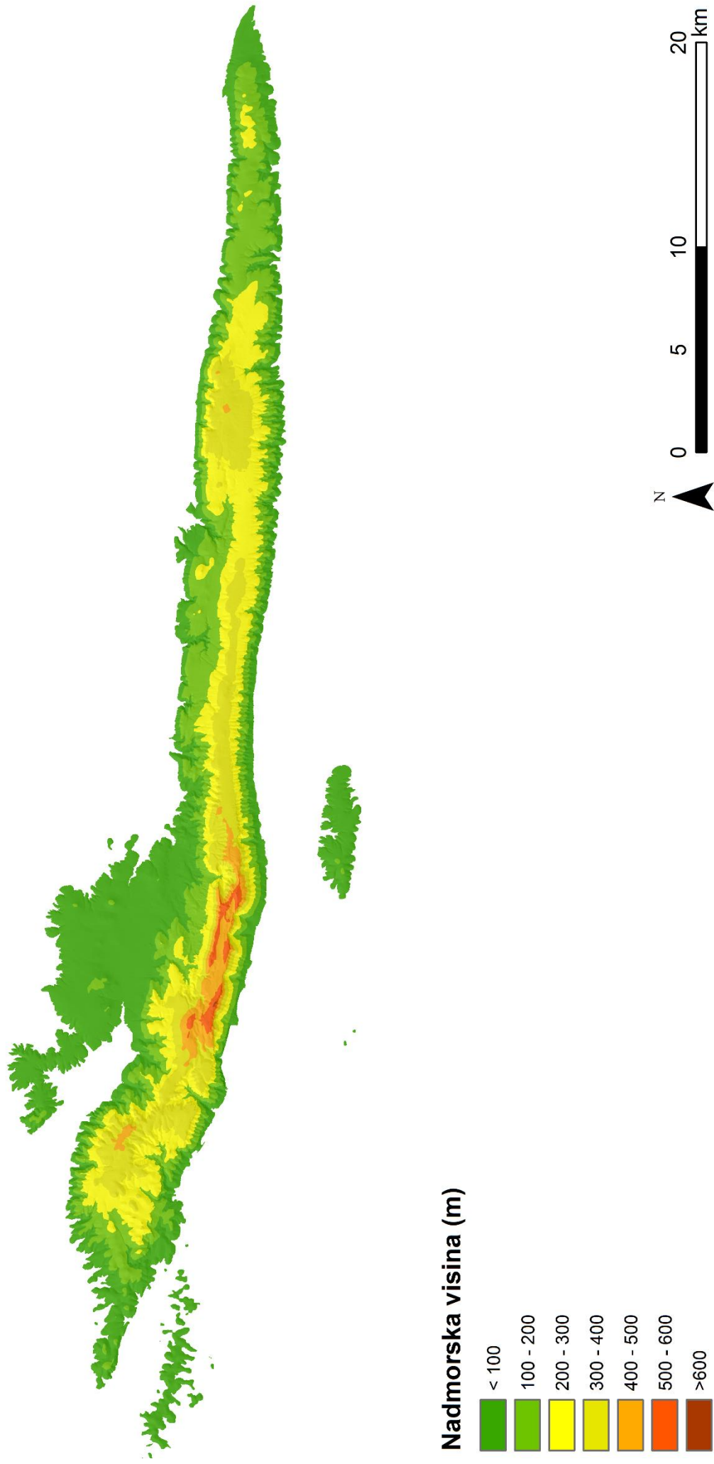
Sl. 5. Hipsometrijska karta otoka Hvara
