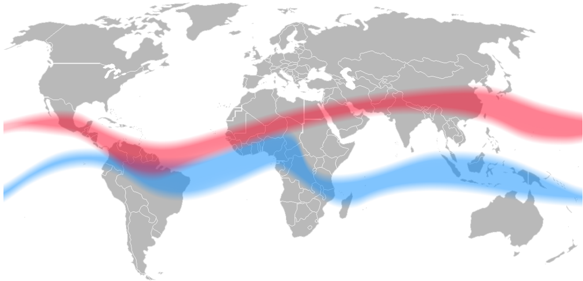
Slika 1.8. Shematski prikaz položaja ITCZ-a u siječnju (plava linija) i u srpnju (crvena linija). Preuzeto s: https://commons.wikimedia.org/wiki/File:ITCZ_january_july.png .
