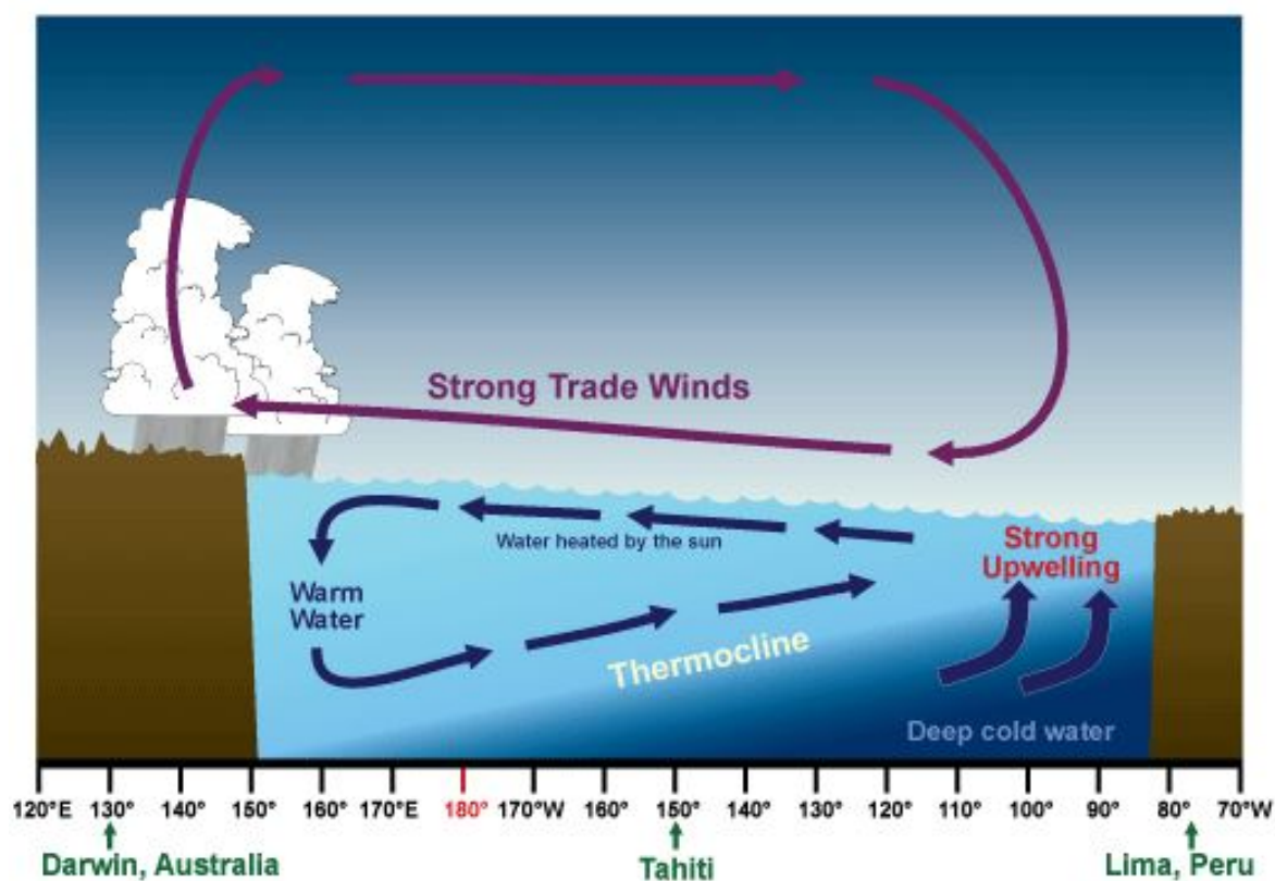
Slika 1.4. Shematski prikaz La Niña faze ENSO-a i njezinog utjecaja. Preuzeto s: https://www.weather.gov/jetstream/enso_patterns .
