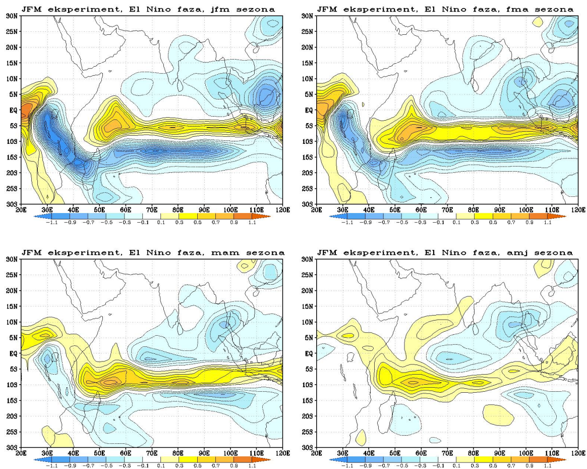
Slika B9. Anomalije oborine nakon jakih El Niño događaja dobivene eksperimentom JFM. Na slikama su redom prikazane prve 4 sezone (u naslovu slike je oznaka sezone).
