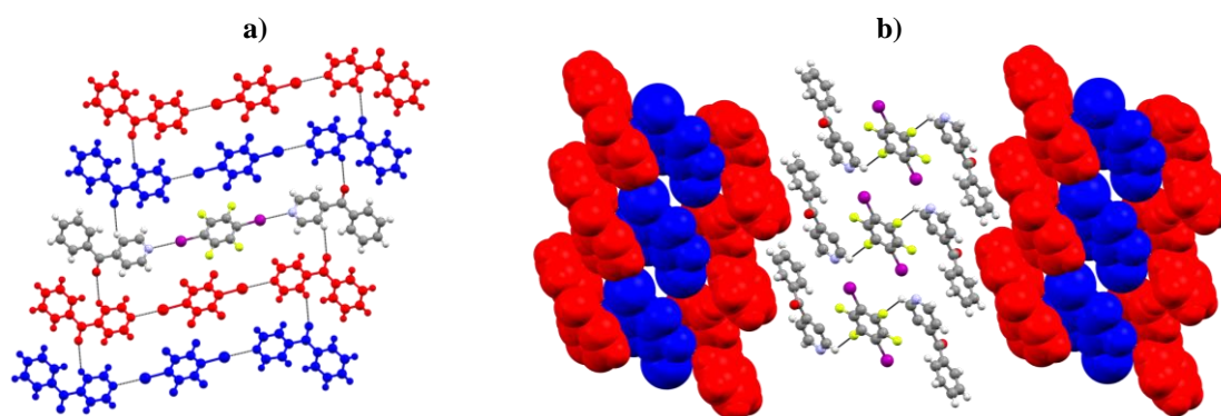
Slika 20. a) Prikaz povezivanja trimera (4\text{bzpy})_2(14\text{tfib}) u 2D mreže kontaktima \text{C-H}\cdots\text{O} i b) prikaz slaganja 2D mreža u 3D mreže kontaktima \text{C-H}\cdots\text{F} .
