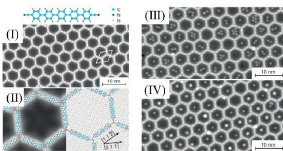
Slika 18. Primjena metalo-organskih koordiniranih nanostrukture kao kvantnih kutija. a) STM slika (\text{NC-Ph}_3\text{-CN})_3\text{Cu}_2 nanoporozne mreže. b) STM slika visoke razlučivosti nanostrukture i usporedba sa strukturnim modelom. c) STM slika željezovih atoma smještenih u šupljine rešetke. d) STM slika željezovih klastera nakon zagrijavanja (preuzeto iz Q. Shen, H. Y. Gao, H. Fuchs, Nano Today 13 (2017) 77–96.)
