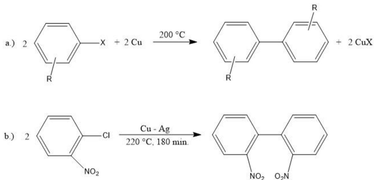
Slika 5. a) Shema Ullmannovog sprezanja između dva halogenirana arila pomoću bakra i b) reakcija sprezanja 1-klor-2-nitrobenzena pomoću Cu-Ag legure
