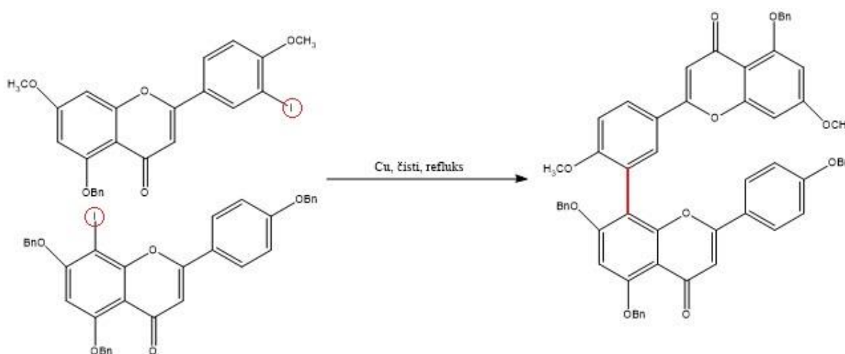
Slika 6. Primjer sinteze biflavanoida pomoću reakcije Ullmannovog sprezanja
