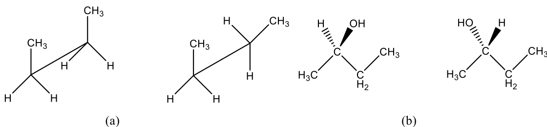
Slika 6. Primjeri konformacijskih (a) i konfiguracijskih (b) izomera.
