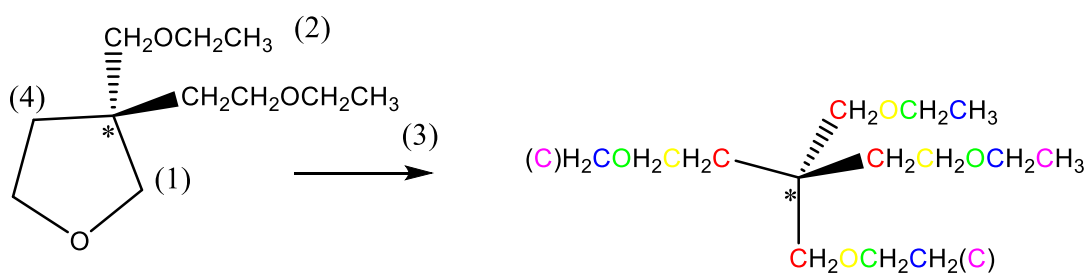
Slika 13. Određivanje prioriteta kiralnog središta u cikličkoj molekuli.
