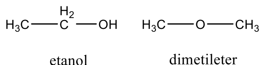
Slika 5. Primjeri konstitucijskih izomera molekulske formule \text{C}_2\text{H}_6\text{O} .
