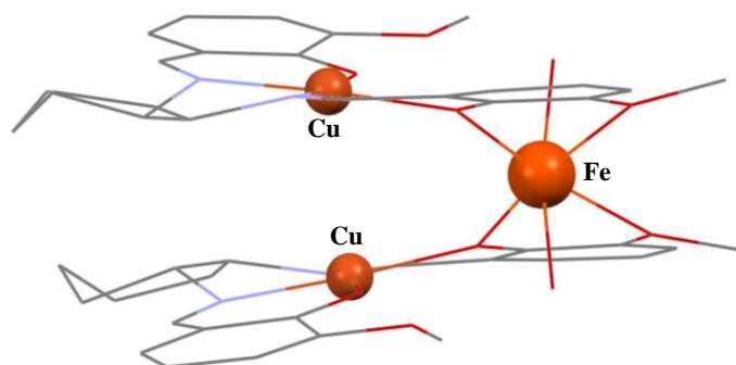
Slika 4. Diskretna jedinica heterometalnog trinuklearnog [Cu 2 Fe] spoja ( YUVREN ). Tamnonarančastom bojom označen je bakrov atom, narančastom željezov atom, crvenom kisikov atom i svijetloplavom dušikov atom. Protuion, molekule otapala te vodikovi atomi uklonjeni su radi preglednosti.
