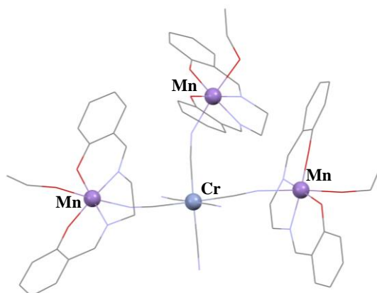
Slika 17. Heterometalni trinuklearni grozd [\text{Mn}_3\text{Cr}] ( CASZEC ). Sivom bojom označen je kromov atom, ljubičastom manganovi atomi, crvenom kisikovi atomi te svjetloplavom dušikovi atomi. U aksijalnom položaju nalaze se koordinirane molekule etanola. Molekule otapala te vodikovi atomi uklonjeni su radi preglednosti.
