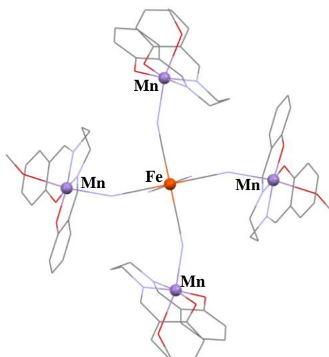
Slika 18. Heterometalni pentanuklearni grozd [\text{Mn}_4\text{Fe}] ( IKERAR ). Žutom bojom označen je željezov atom, ljubičastom manganovi atomi, crvenom kisikovi atomi te svjetloplavom dušikovi atomi. Protuion, vodikovi atomi uklonjeni su radi preglednosti.
