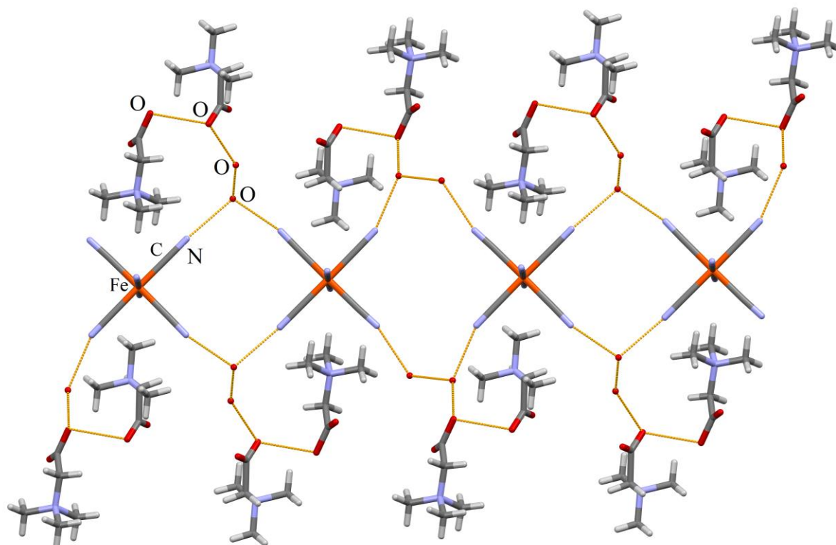
Slika 5. Struktura betainijevog heksacijanoferata(III) tetrahidrata, vodikove veze prikazane su narančastim crticama. Vodikovi atomi na molekulama vode nisu prikazani radi preglednosti. 37
