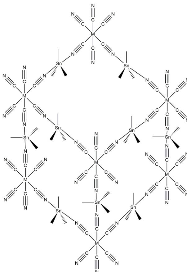
Slika 4. Idealizirana struktura super-berlinskog modrila sa [\text{Me}_3\text{Sn}]^+ kao protuionom
