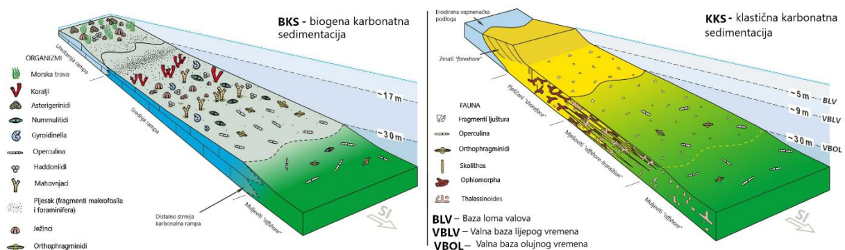
Slika 25. Shematski paleoekološki modeli za biogenenu karbonatnu sedimentaciju (BCS) i klastičnu karbonatnu sedimentaciju (CCS) na antiklinalnim izdignućima (preuzeto i modificirano prema Ćosović et al., 2018).
