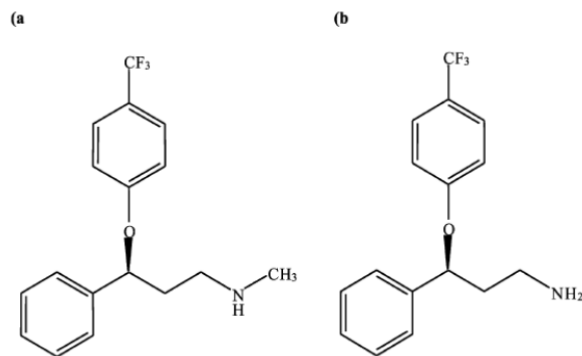
Slika 2. Strukturna formula a) fluoksetina i b) norfluoksetina
