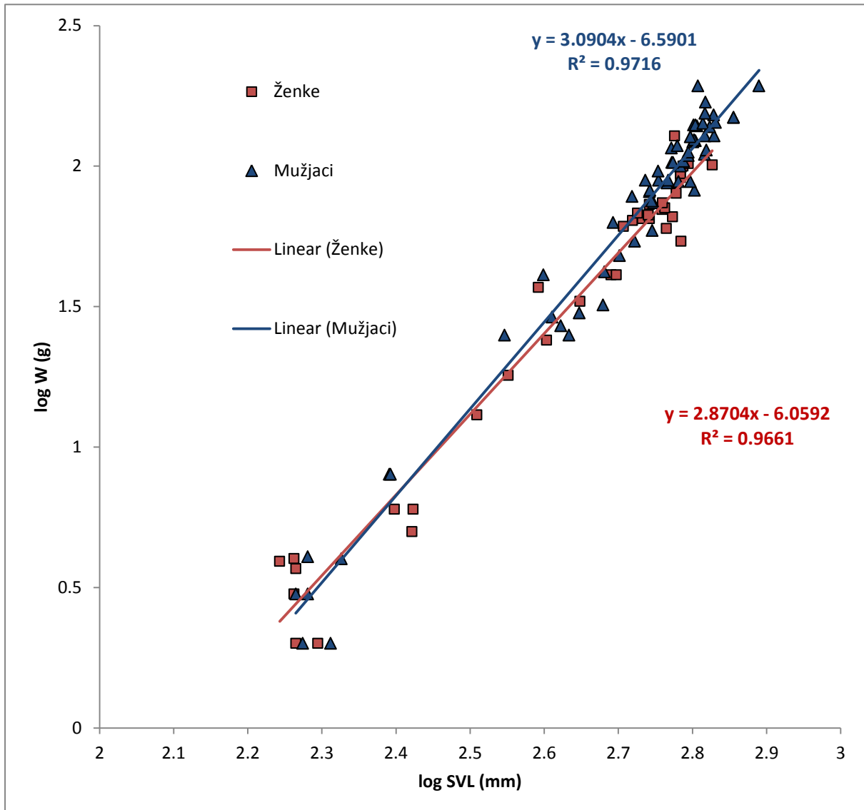
Slika 10. Jednofaktorska ANCOVA logaritmiranih vrijednosti standardne duljine tijela (SVL) i težine (W) vrste H. gemonensis , F = 6.723 , p = 0.011
