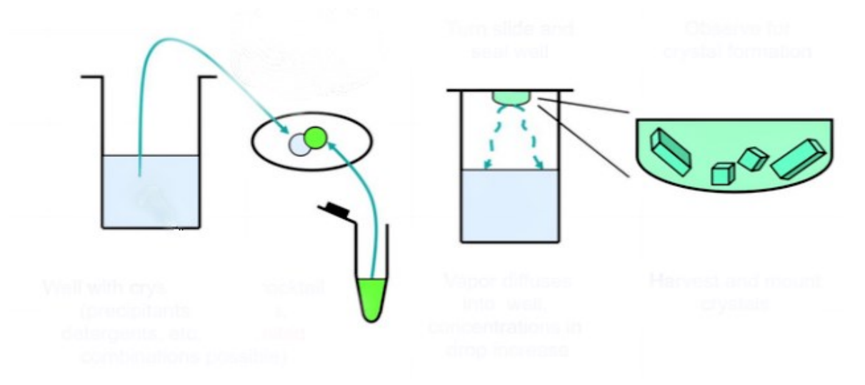
Slika 15. Postupak kristalizacije metodom difuzije para viseće kapi.
