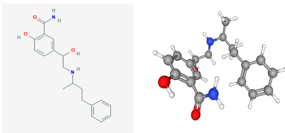
Slika 9. Prikaz dvodimenzijske strukture labetalola te prikaz modelom kuglice i štapića (sivo obojani su atomi ugljika, plavo dušika, a crveno kisika) 15
