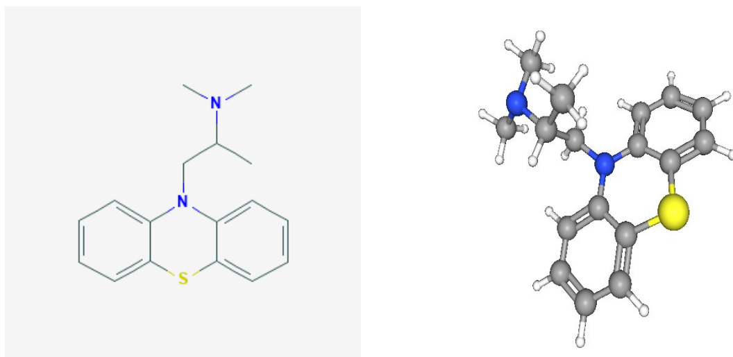
Slika 8. Prikaz molekule prometazina te prikaz modelom kuglice i štapića (sivo su obojani atomi ugljika, plavo obojeni atomi dušika, a žuto je obojen atom sumpora) 14
