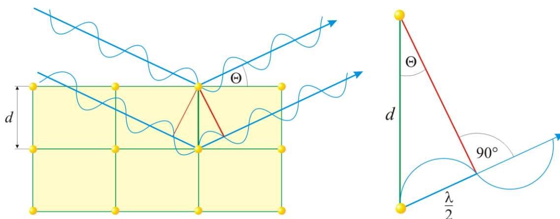
Slika 13. Braggov zakon
