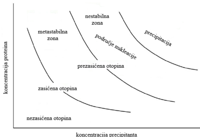
Slika 10. Shematski prikaz krivulje topljivosti proteina kao funkcije ovisnosti koncentracije precipitanta i koncentracije proteina
