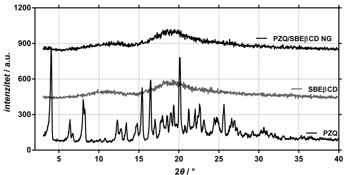
Slika 39. XRPD uzorak PZQ-a, sulfobutil- \beta -ciklodekstrina ( \text{SBE}\beta\text{CD} ) i njihov ekvimolarni mljeveni produkt pripremljen suhim mljevenjem (NG).
