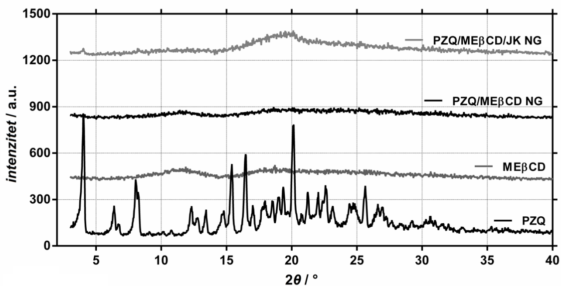
Slika 38. XRPD uzorak PZQ-a, metil- \beta -ciklodekstrina ( \text{ME}\beta\text{CD} ) i njihov ekvimolarni mljeveni produkt pripremljen suhim mljevenjem (NG).
