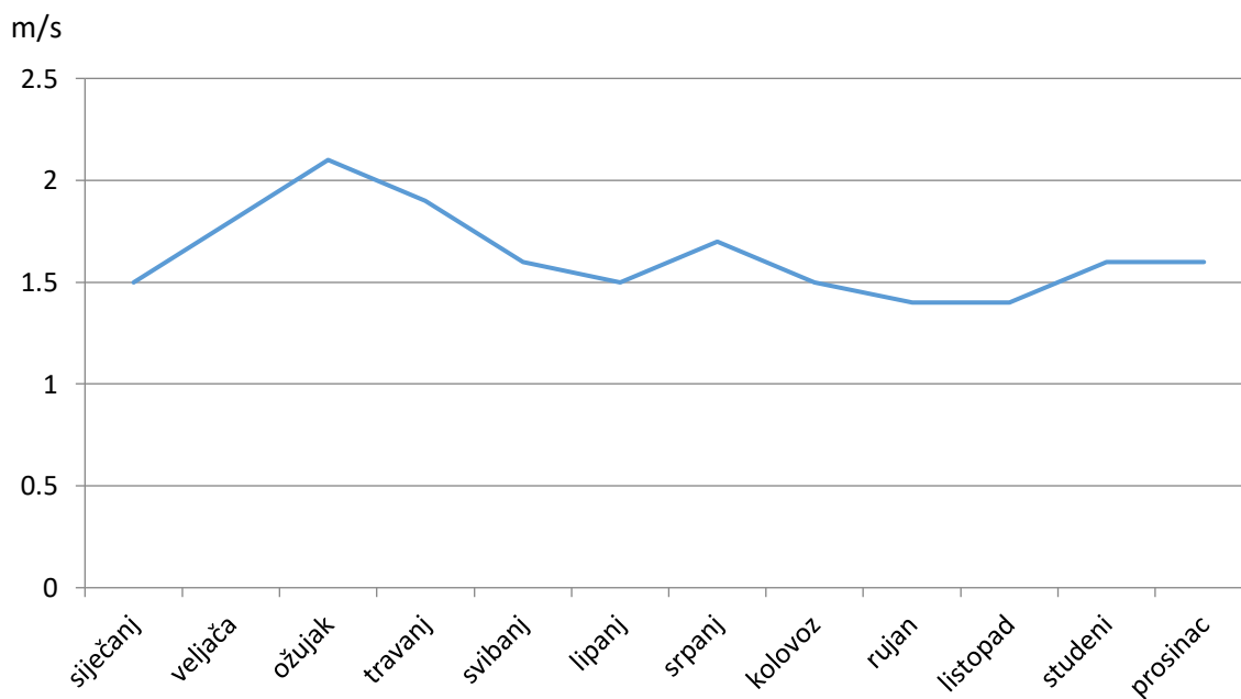
Sl. 8: Godišnji hod srednjih mjesečnih brzina vjetra u Sinju za razdoblje 1981.-2010.
