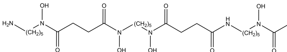
Slika 9. Desferioksamin B
