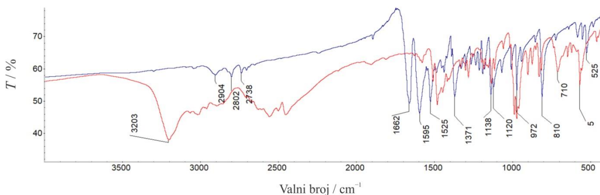
Slika 21. FTIR spektri reakcijske smjese spoja C (plavi spektar), te spoja C , hidroksilamonijevog klorida i katalitičke količine etanola (crveni spektar) nakon 30 minuta mljevenja.
