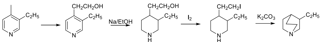
Shema 1. Sinteza 3-etilkinuklidina.
