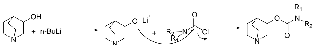
Shema 44. Sinteza karbamata upotrebom n -butillitija kao baze.
