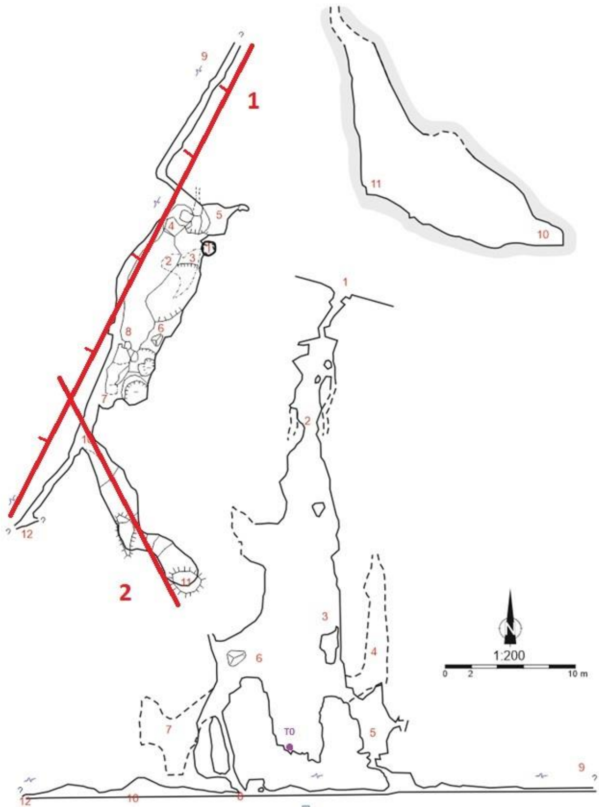
Sl. 25. Digitalizirani nacrt Velebitaške jame na temelju nacrt iz 1973. godine (Izradio: M. Čepelak, digitalizirala: T. Selaković) s dodatim prikazom pružanja pukotinskih sustava (1, 2) i s točkom mjerenja mikroklimae, radona i CO 2 (T0)
