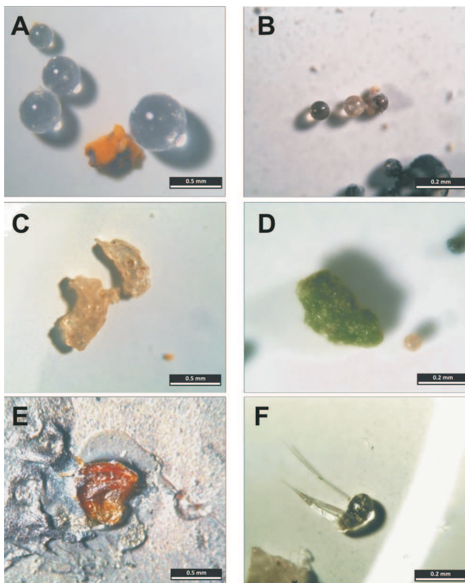
Slika 3.6. Mikrouzorci eocenske starosti: A) staklene sferule i žuti matiks, B) crne sferule, C) vesikularna stakla, D) zeleno mineralno zrno, E) narančasto mineralno zrno i F) mikrotektit
