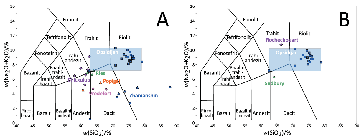
Slika 2.4. Usporedba sastava opSIDijana i impaktnih stakala A) iz tablice 3 i B) iz tablice 4
