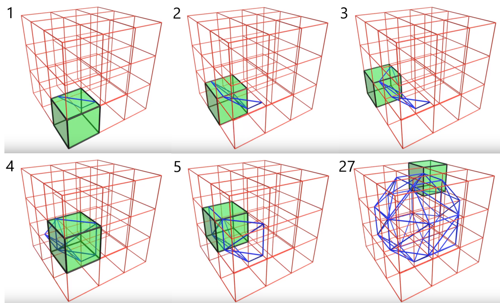
Slika 4.5: Slikoviti prikaz marching cubes algoritma 1
