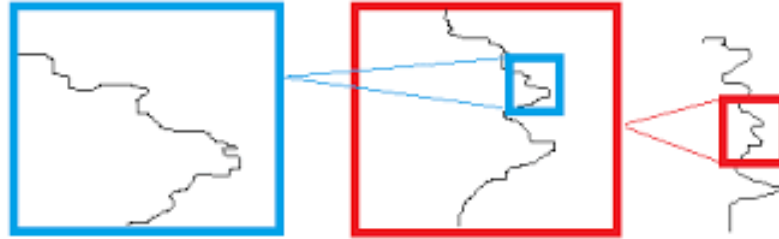
Slika 3.1: Samosličnost obale
