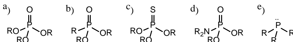
Slika 6. Organofosforovi spojevi a) fosfatni esteri; b) fosfonatni esteri; c) tiofosfatni esteri; d) fosforamidati; e) fosfini
