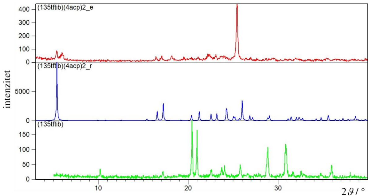
Slika D65. Usporedba difraktograma polikristalnog uzorka kokristala (135\text{tfib})(4\text{acp})_2 dobivenog mljevenjem ( (135\text{tfib})(4\text{acp})_2\text{_e} ) s difraktogramom generiranim iz kristalne strukture ( (135\text{tfib})(4\text{acp})_2\text{_r} ) i difraktogramom donora halogenske veze 135\text{tfib} .
