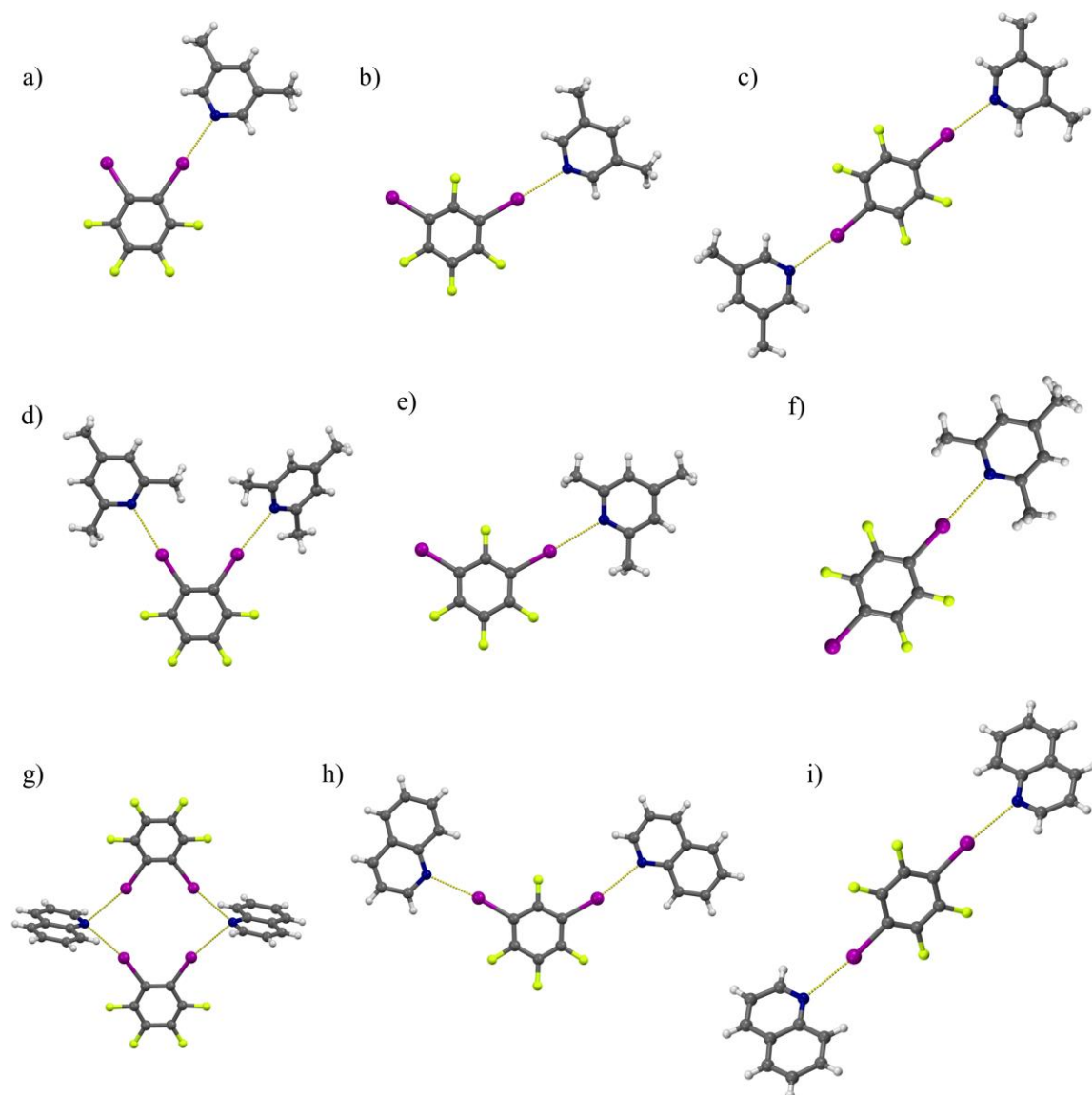
Slika 28. Supramolekulski kompleksi s halogenskim vezama I...N u odabranim kokristalima s ditopičnim donorima: a) (12tfib)(35lut), b) (13tfib)(35lut), c) (14tfib)(35lut) 2 , d) (12tfib)(246kol) 2 , e) (13tfib)(246kol), f) (14tfib)(246kol), g) (12tfib)(kin), h) (13tfib)(kin) 2 , i) (14tfib)(kin) 2 .
