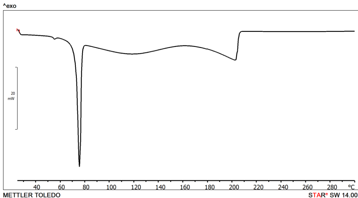
Slika D83. Termogram razlikovne pretražne kalorimetrije kokristala (14tfib)(2pik)_2 dobivenog mljevenjem reaktanata.
