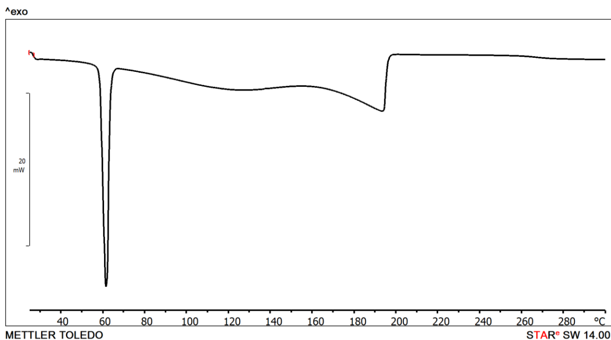
Slika D84. Termogram razlikovne pretražne kalorimetrije kokristala (14tfib)(3pik)_2 dobivenog mljevenjem reaktanata.
