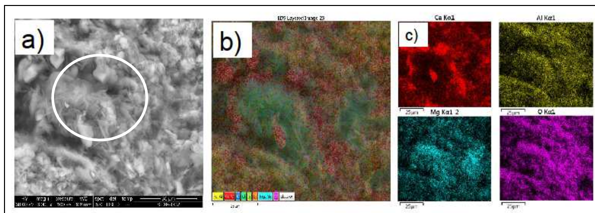
Slika 23. SEM BSED snimak: (a) elementna mapa, (b) pore uzorka S-DTGLO2 i mape kalcija, aluminija, magnezija i kisika (c)
