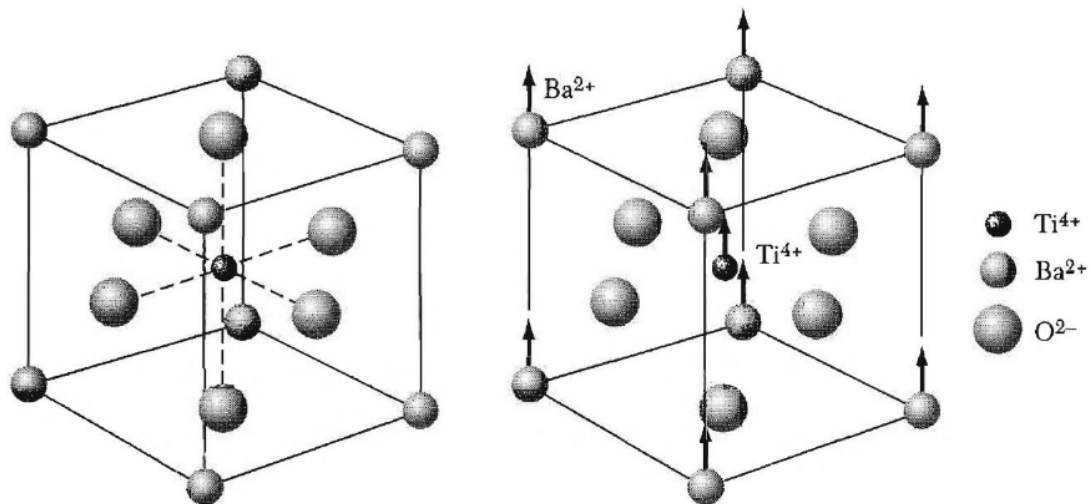
Slika 3.4: Struktura \text{BaTiO}_3 . Struktura (lijevo) je kubična s ionima \text{Ba}^{2+} u kutevima, \text{O}^{2-} ionima na licima, te \text{Ti}^{4+} ionima u središtu. Ispod kritične temperature T_C , ioni \text{Ba}^{2+} i \text{Ti}^{4+} pomiču se u odnosu na ione \text{O}^{2-} te se razvija dipolni moment (desno). Slika preuzeta iz [10]
