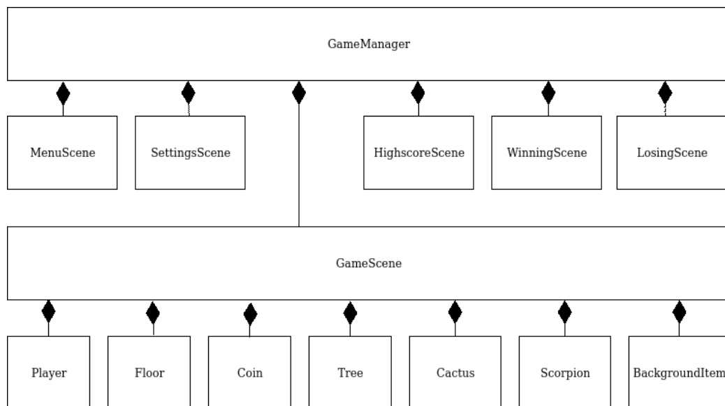
Slika 3.7: Class dijagram
