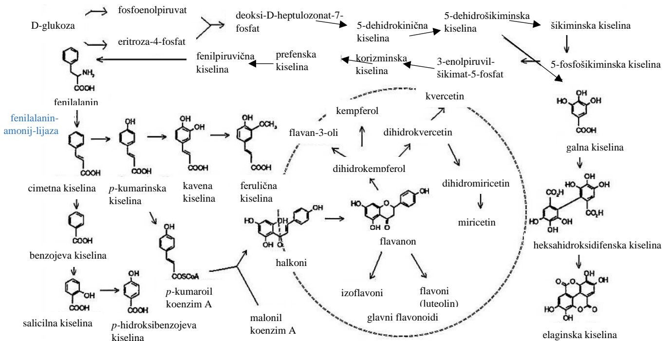
Slika 4. Biosintetski put fenilpropanoida. Preuzeto i prilagođeno prema Mandal i sur. (2010).
