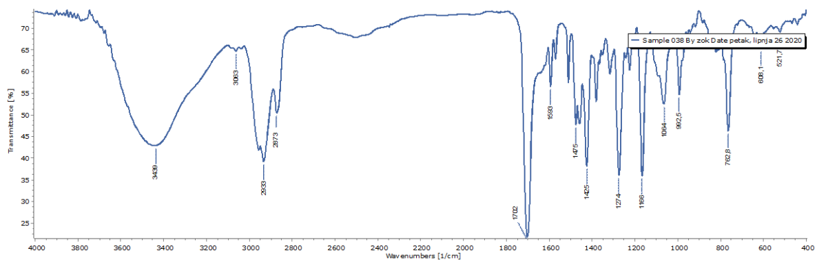
Slika D12. IR spektar spoja 4
