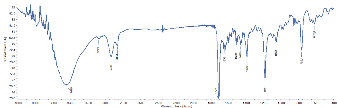
Slika D23. IR spektar spoja 7
