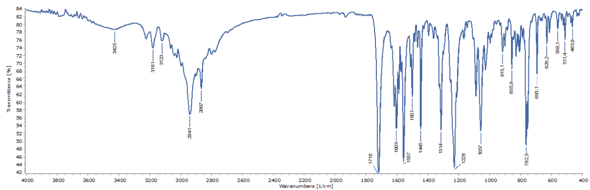
Slika D18. IR spektar spoja 6
