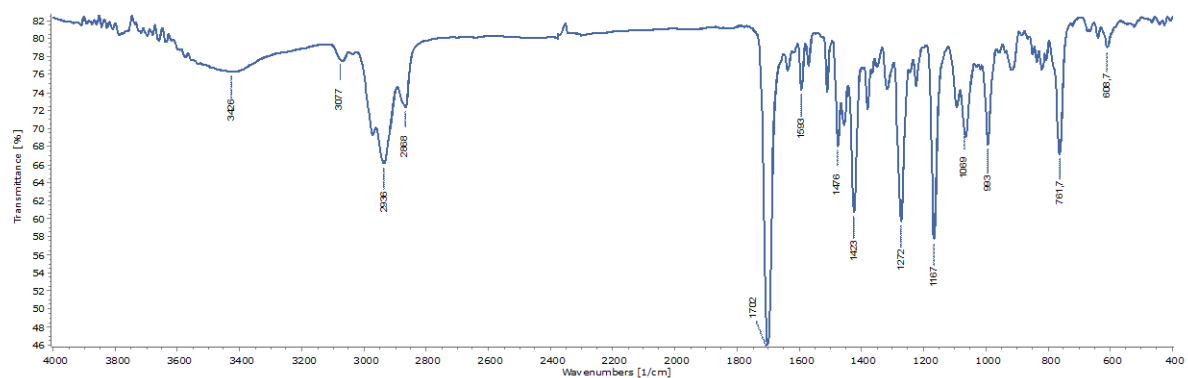
Slika D26. IR spektar spoja 8
