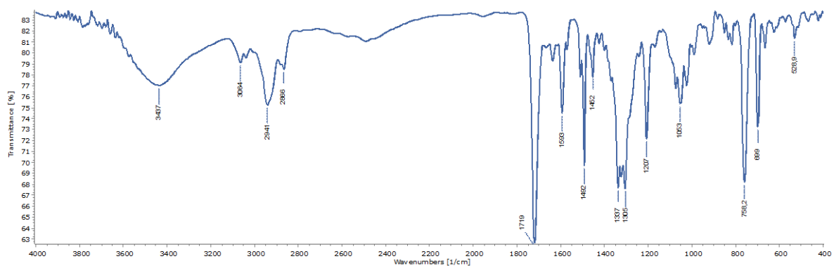
Slika D29. IR spektar spoja 9
