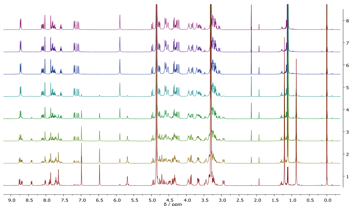
Slika 11. Titracija ^1\text{H} NMR spoja L ( c = 1,42 \times 10^{-3} \text{ mol dm}^{-3} ) s natrijevim perkloratom ( c = 2,45 \times 10^{-2} \text{ mol dm}^{-3} ) u MeOD pri 25 °C.
