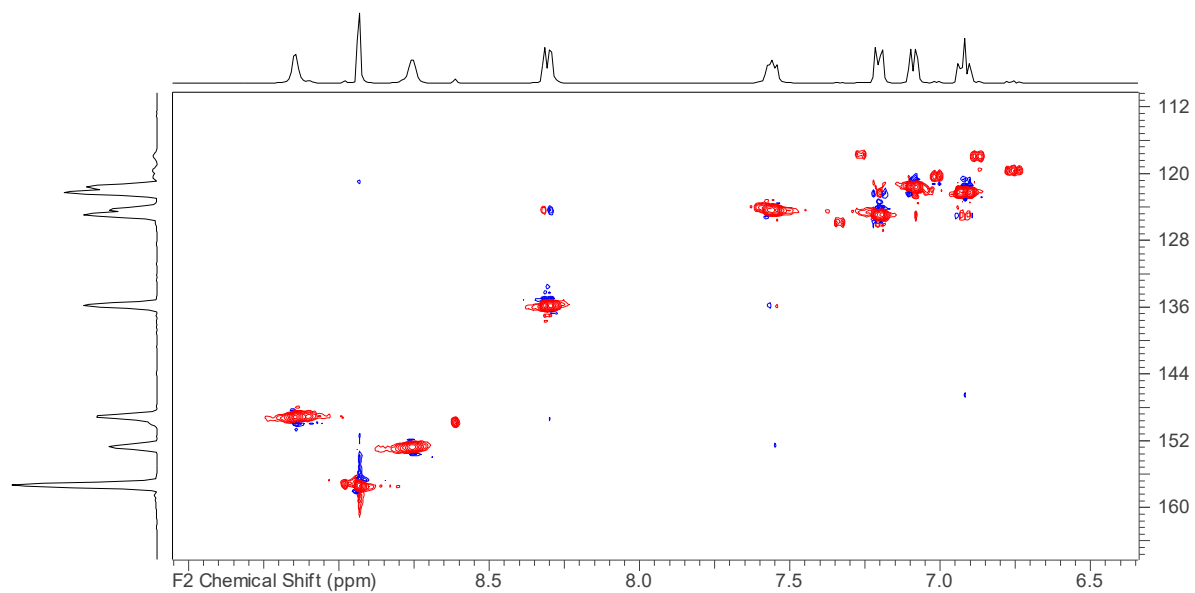
Slika D31. Uvećani prikaz HMBC spektra 4 · aceton
