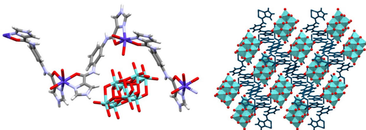
Slika 17. \{[CoL(H_2O)_2]_2[Mo_8O_{26}]\}_n ( A ). Lijevo je prikaz soli građene od koordinacijskog polimera i oktamolibdata, a desno njeno pakiranje duž kristalografske osi b . Atomi vodik koordinirane vode nisu prikazani.
