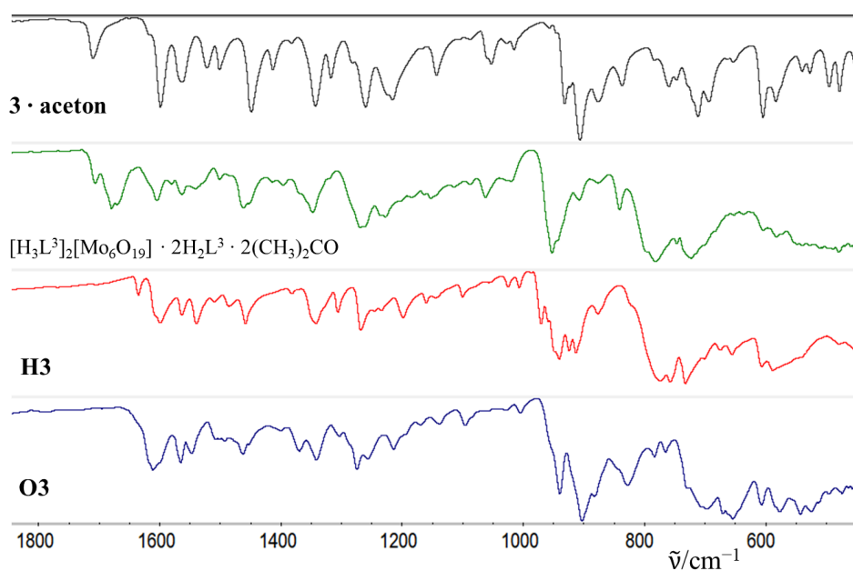
Slika 42. Uvećani prikaz usporedbe IR spektara svih spojeva nastalih reakcijom s ligandom H 2 L 3 .
