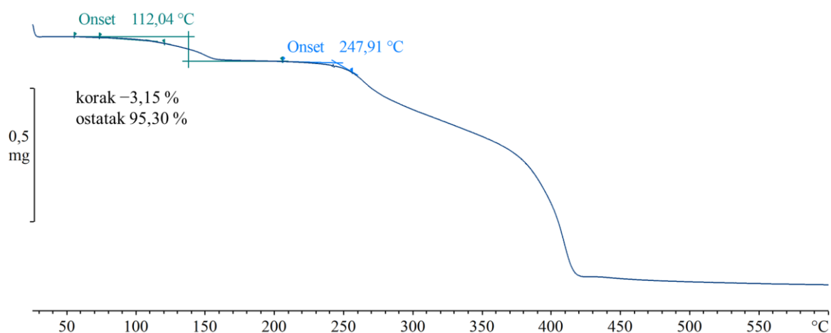
Slika 43. Termogram raspada O2 . Pad mase na početku mjerenja (ispod 50 °C) pripisan je nedovoljnoj posušenosti uzorka zbog kojeg je zbroj postotaka pada mase u prvom koraku i ostatka manji od 100 %.
