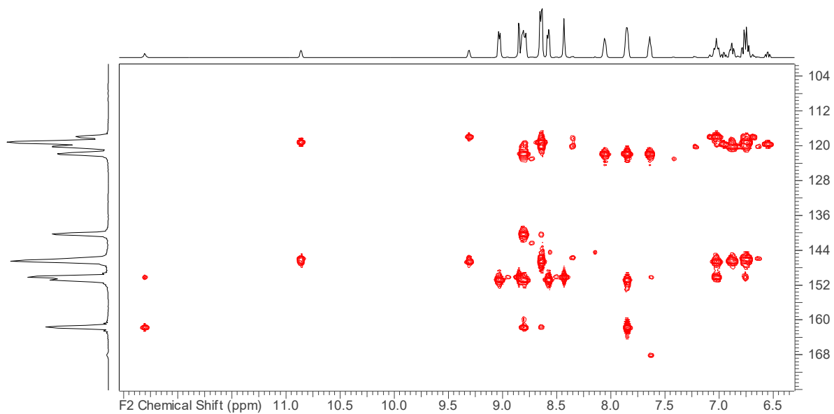
Slika D20. Uvećani prikaz HMBC spektra H 2 L 3
