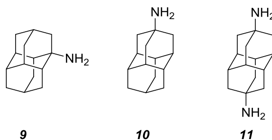
Slika 16. Struktureaminskih spojeva 9-11
