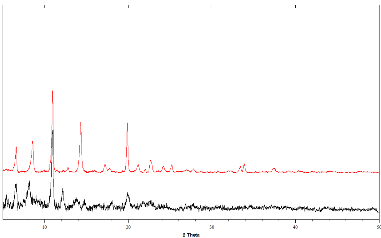
Slika D47. Usporedba difraktograma praha kompleksnog spoja [\text{MoO}_2(\text{H}_2\text{T})]_n , dobivenog reakcijom u acetonu (crno) i acetonitrilu (crveno)
