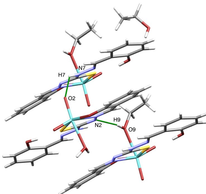
Slika D58. Prikaz graf-set motiva C_2^2(12) u kristalnoj strukturi kompleksnog spoja [\text{MoO}_2(\text{H}_2\text{T})(\text{EtOH})][\text{MoO}_2(\text{H}_2\text{T})(\text{H}_2\text{O})] \cdot \text{EtOH} . Vodikove veze prikazane su zelenom bojom
