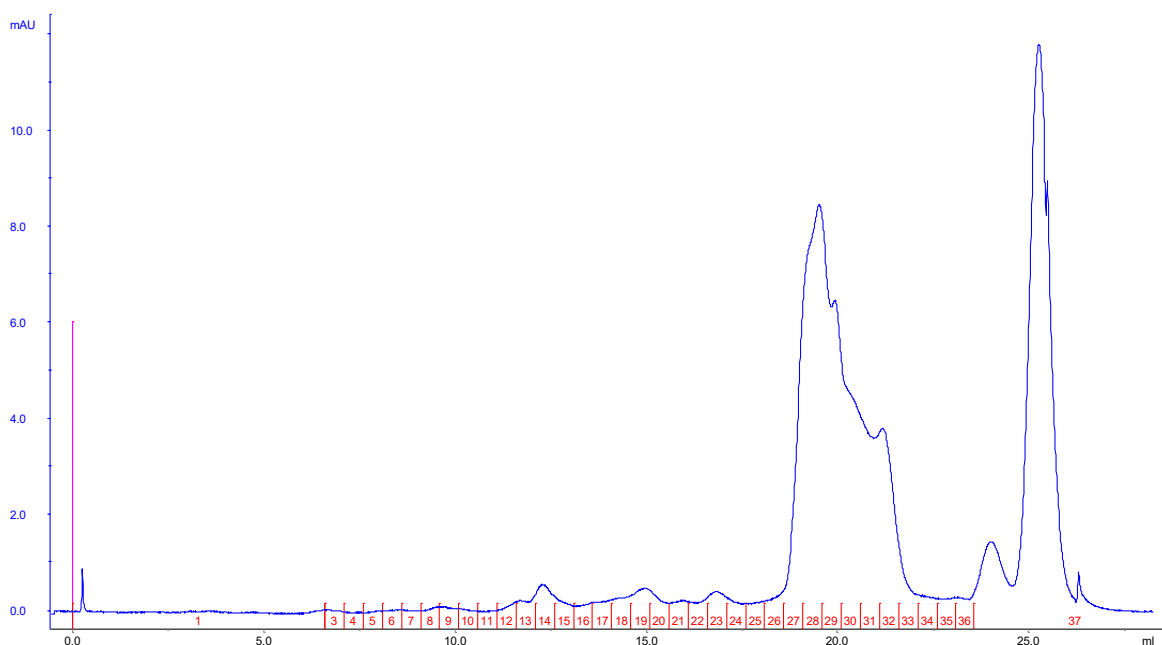
Slika 33. Kromatogram DRG1 proteina dobiven gel-filtracijom na uređaju ÄKTA-FPLC uz Superdex TM 200 Increase 10/300 GL kolonu i protok 1,0 \text{ mL min}^{-1} . Na kolonu je nanoseno 120 \mu\text{L} uzorka. Pufer za eluciju sadržavao je 25 \text{ mmol/L} Tris-HCl (pH 7,5), 150 \text{ mmol/L} NaCl. Plava linija označava propušteni uzorak proteina DRG1, a crvenom bojom označene su frakcije.
