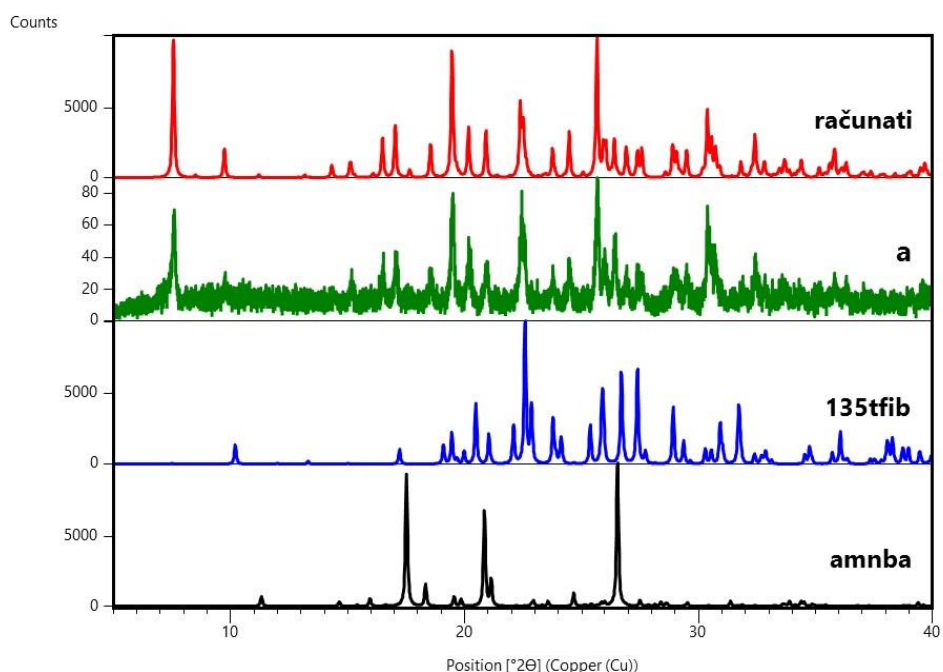
Slika D19. Usporedba difraktograma praha produkta kristalizacijskog pokusa priređivanja jediničnog kristala kokristala (\text{amnba})(135\text{tfib})_2 iz jednog otapala s difraktogramom praha amnba , 135tfib i difraktograma računatog iz podataka dobivenih difrakcijom rentgenskog zračenja na jediničnom kristalu kokristala (\text{amnba})(135\text{tfib})_2 ; a) MeOH (1:1)
