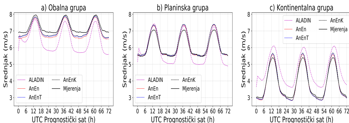
Slika 5.4. Ovisnost srednjaka brzine udara vjetra o prognostičkom satu (UTC) svih prognoza i mjerenja za obalnu (a), planinsku (b) i kontinentalnu (c) grupu postaja u 2018. godini.
