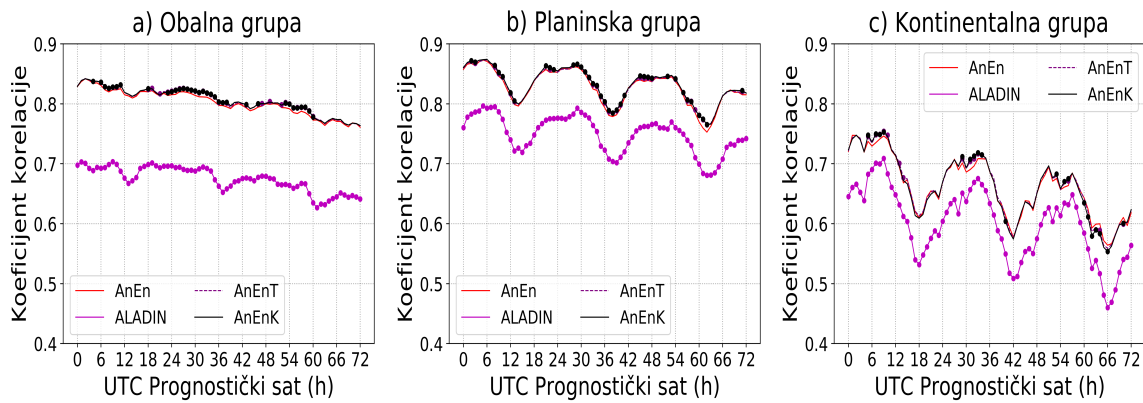
Slika 5.3. Ovisnost koeficijenta korelacije o prognostičkom satu (UTC) svih prognoza za obalnu (a), planinsku (b) i kontinentalnu (c) grupu postaja u 2018. godini. Kružnim markerima označene su vrijednosti koje se značajno razlikuju od prognoze AnEn.
