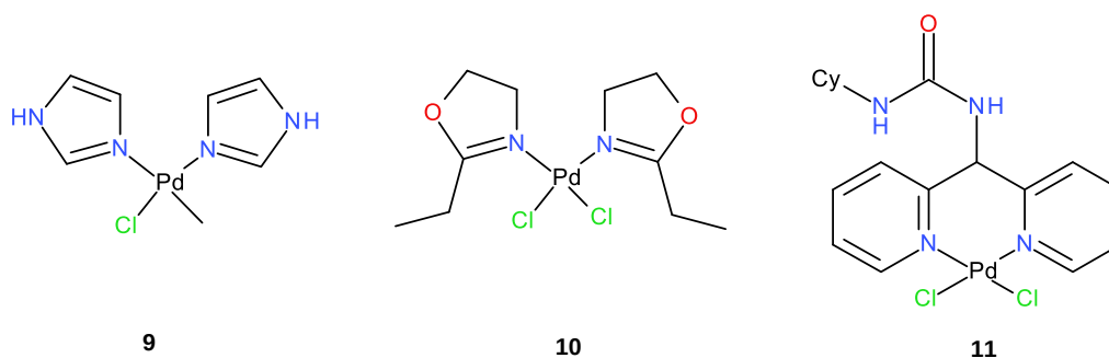
Slika 10. Strukturne formule molekula paladij-dušik kompleksa kao katalizatora 36,37,38,39
