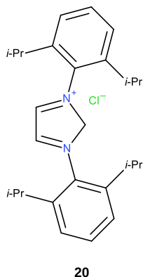
Slika 16. Strukturna formula bis-2,6-diizopropilfenildihidroimidazolijskoga klorida
