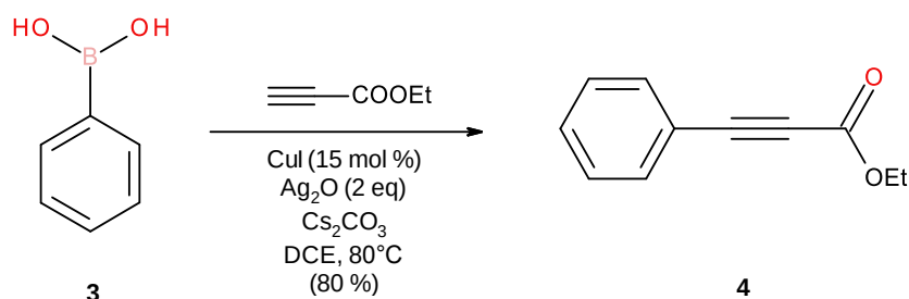
Slika 6. Shematski prikaz bakrom i srebrom ko-katalizirana Sonogashira reakcije bez dodatka liganada 30
