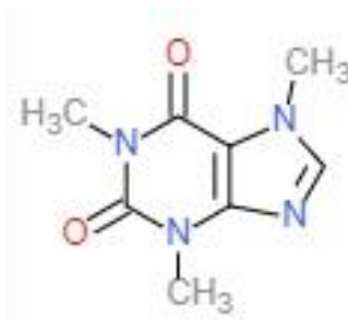
Slika 2.8. Molekulska struktura kofeina.
