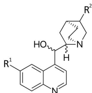
Slika 2. Struktura kinina
