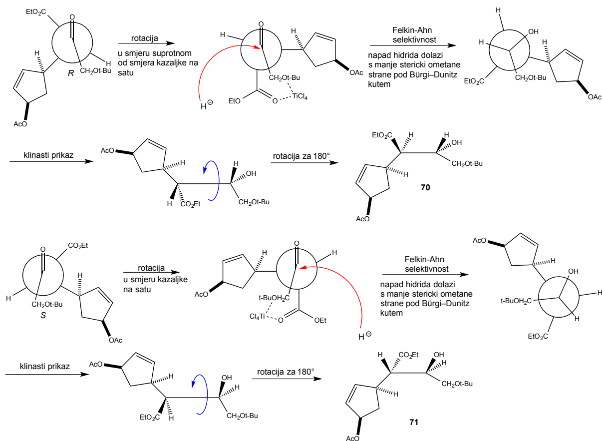
Slika 22. Objašnjenje stereokemijskog ishoda anti redukcije stereoisomera 69 Felkin-Ahn modelom
