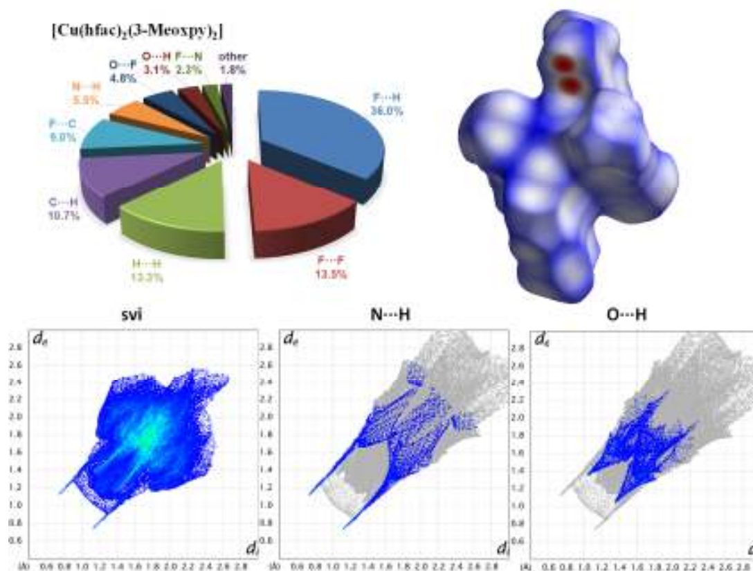
Slika 20. Udjeli najznačajnijih kontakata za [\text{Cu}(\text{hfac})_2(3\text{-Meoxy})_2] (gore lijevo). Hirshfeldova ploha mapirana s d_{\text{norm}} vrijednostima (gore desno), 2D dijagrami otiska prsta za sve kontakte te zasebno za \text{O}\cdots\text{H} i \text{N}\cdots\text{H} 14
