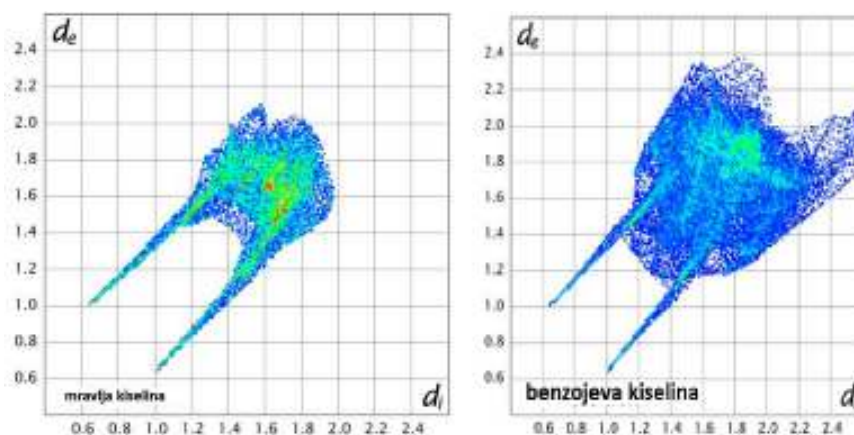
Slika 7. Dijagram otiska prsta za mravlju i benzojevu kiselinu 8
