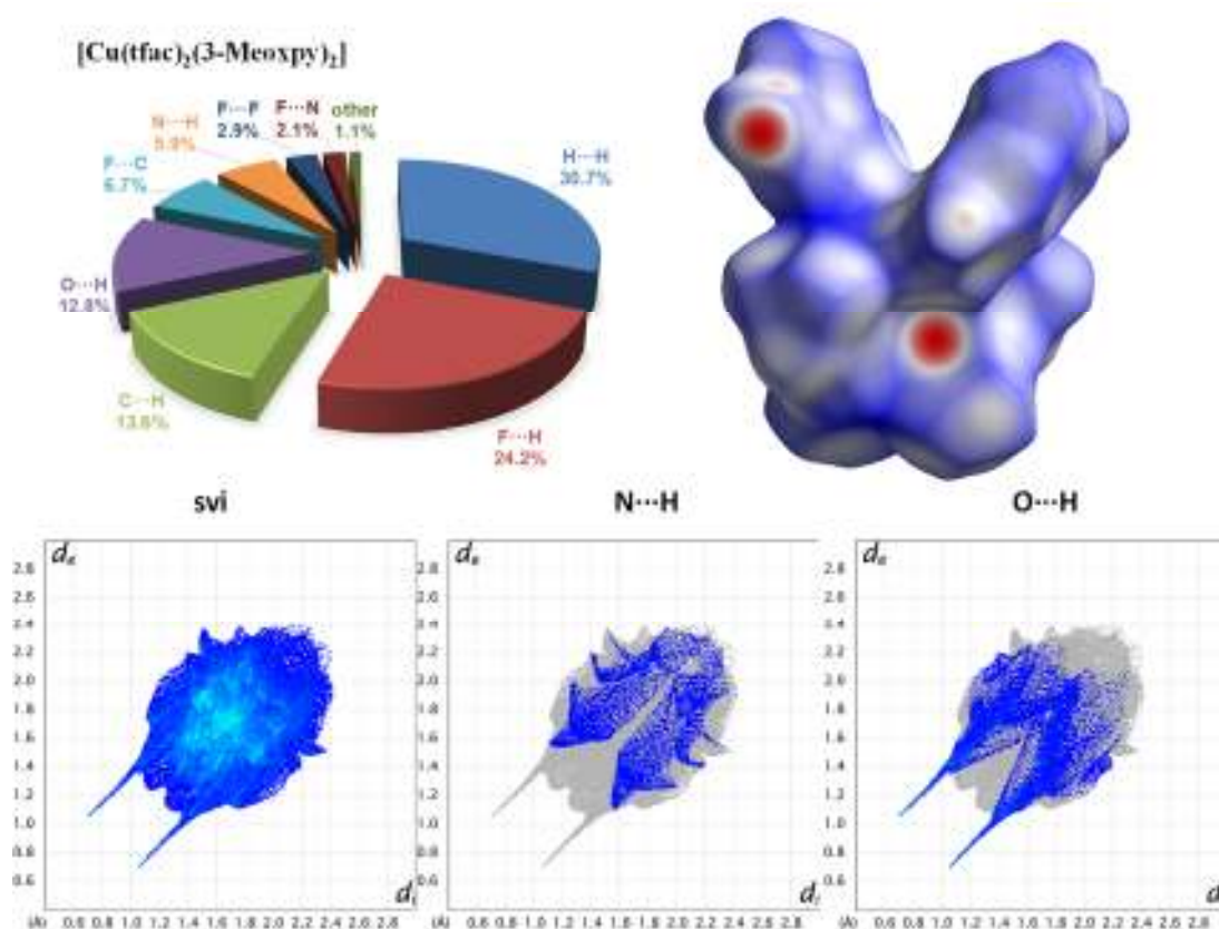
Slika 28. Udjeli najznačajnijih kontakata za [\text{Cu}(\text{tfac})_2(3\text{-Meoxpy})_2] (gore lijevo). Hirshfeldova ploha mapirana s d_{\text{norm}} vrijednostima (gore desno), 2D dijagrami otiska prsta za sve kontakte te zasebno za \text{O}\cdots\text{H} i \text{N}\cdots\text{H} 14
