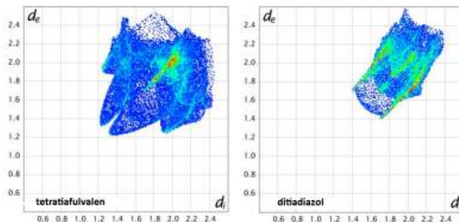
Slika 10. 2D dijagram otiska prsta za tetratriafulvalen i ditiadiazol 8
