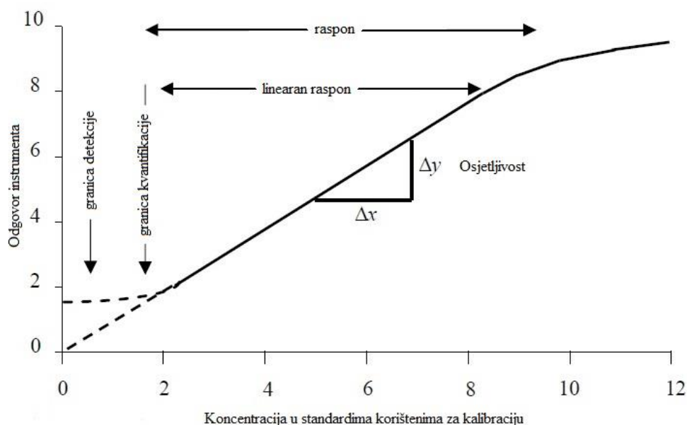
Slika 2. Tipična ovisnost odgovora instrumenta o koncentraciji u standardima korištenim za kalibraciju. Grafički su identificirane sljedeće značajke metode: granica detekcije, granica kvantifikacije, osjetljivost, linearan raspon te raspon 2
