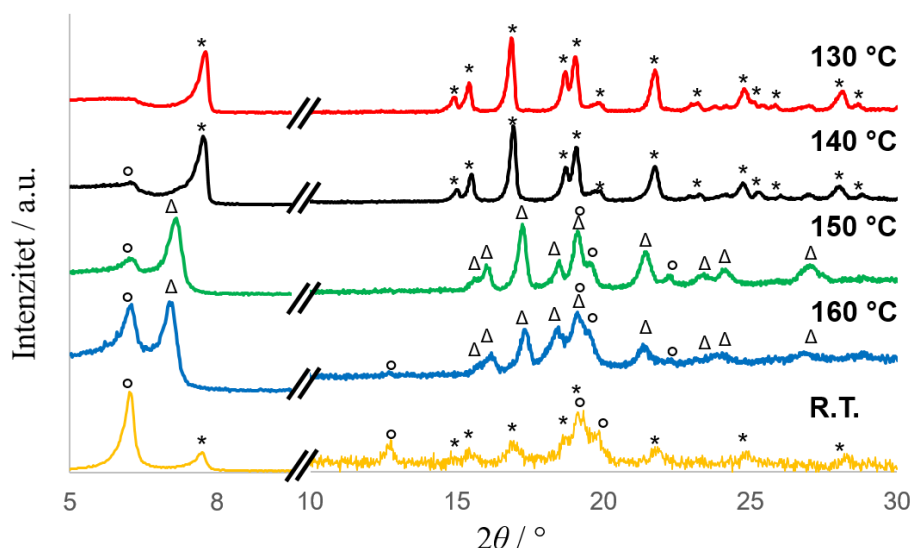
Slika 72. Prikaz temperaturno ovisnih difraktograma praha spoja 7c . Zvezdicom (*) su označeni difrakcijski maksimumi koji odgovaraju spoju 7c , kružićem (○) maksimumi koji odgovaraju spoju 7e , a trokutom (△) maksimumi koji odgovaraju neidentificiranoj fazi. Difraktogrami praha razlomljeni su na dva dijela, 5–10° i 10–30°, i nisu na istoj skali intenziteta.
