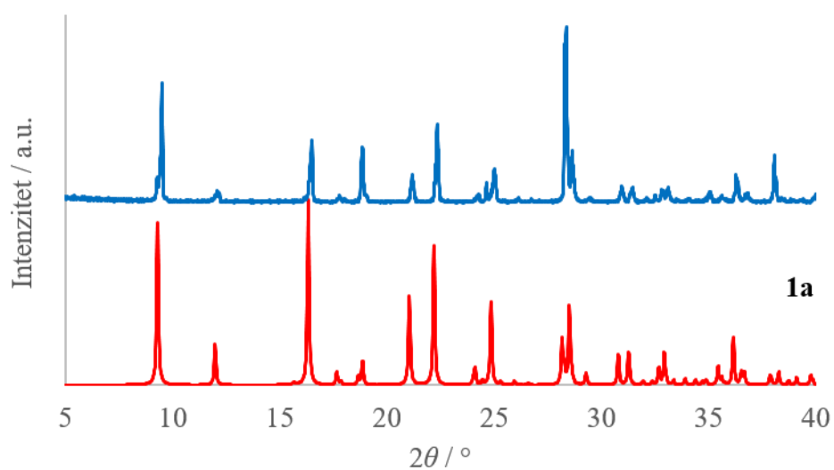
Slika D1. Usporedba difraktograma praha 1a dobivenog iz sinteze (plavo) i difraktograma praha izračunatog iz kristalne strukture 1a (crveno).
