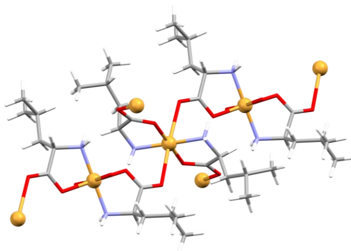
Slika 5. 2D koordinacijski polimer s oktaedarskom geometrijom oko bakrovog(II) atoma u kristalnoj strukturi spoja trans -[Cu( \mu -D-Leu)( \mu -L-Leu)] _n . Atomi bakra(II) prikazani su narančastim kuglicama.
