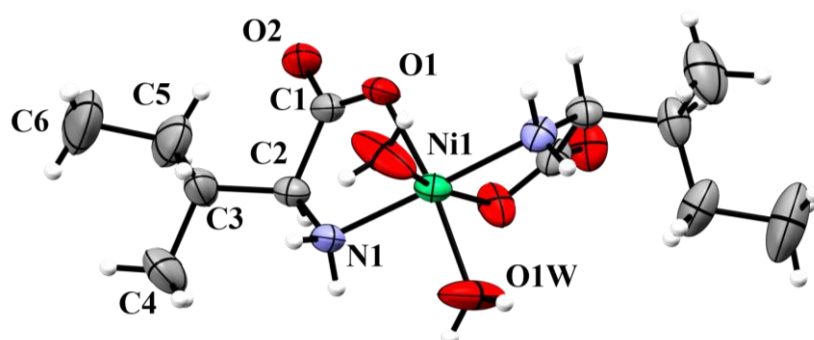
Slika 62. Molekulska struktura spoja 6 sa shemom numeriranja atoma. Vodikovi atomi prikazani su sferama proizvoljnog polumjera, a nevodikovi atomi elipsoidima pomaka, uz razinu vjerojatnosti 50 %.
