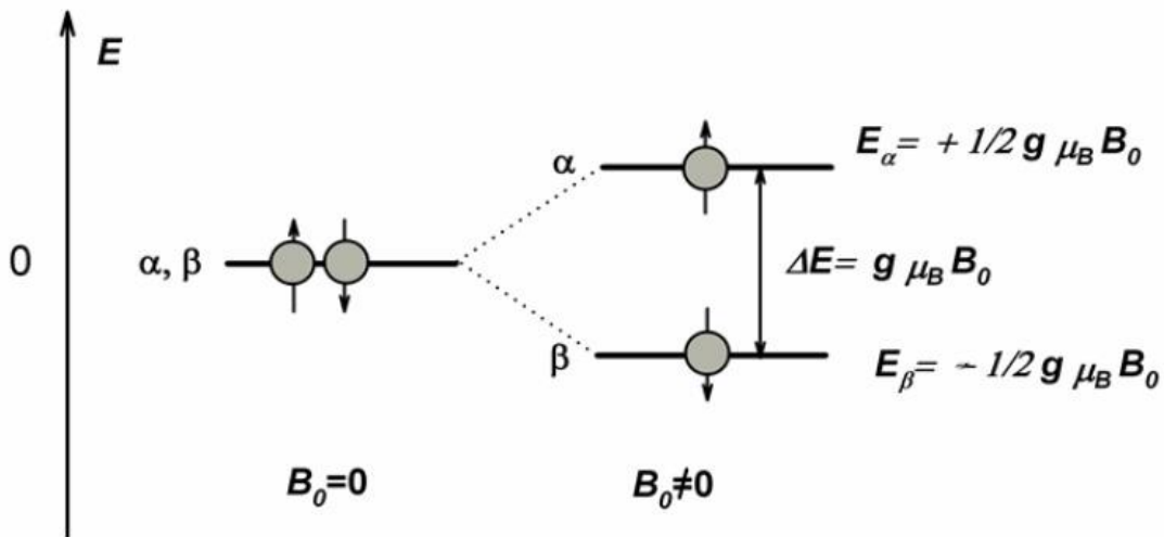
Slika 4.2. Zeemanov efekt – razdvjanje energetske nivoe paramagnetskog sustava u vanjskom magnetskom polju [9]
