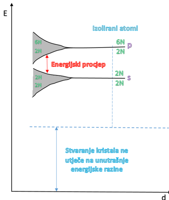
Slika 7.1: Ilustracija kako se energijske razine izoliranih atoma dijele u energijske vrpce kada su atomi na bliskim udaljenostima.
