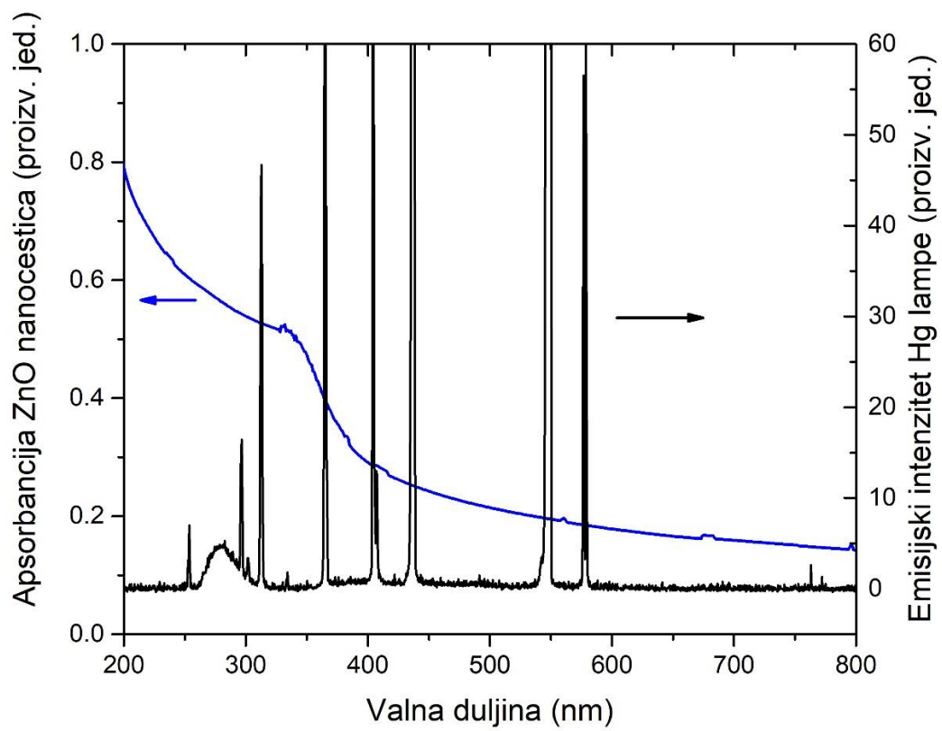
Slika 7 Emisijski intezitet živine lampe zajedno i apsorbancija ZnO nanočestica po valnim duljinama
