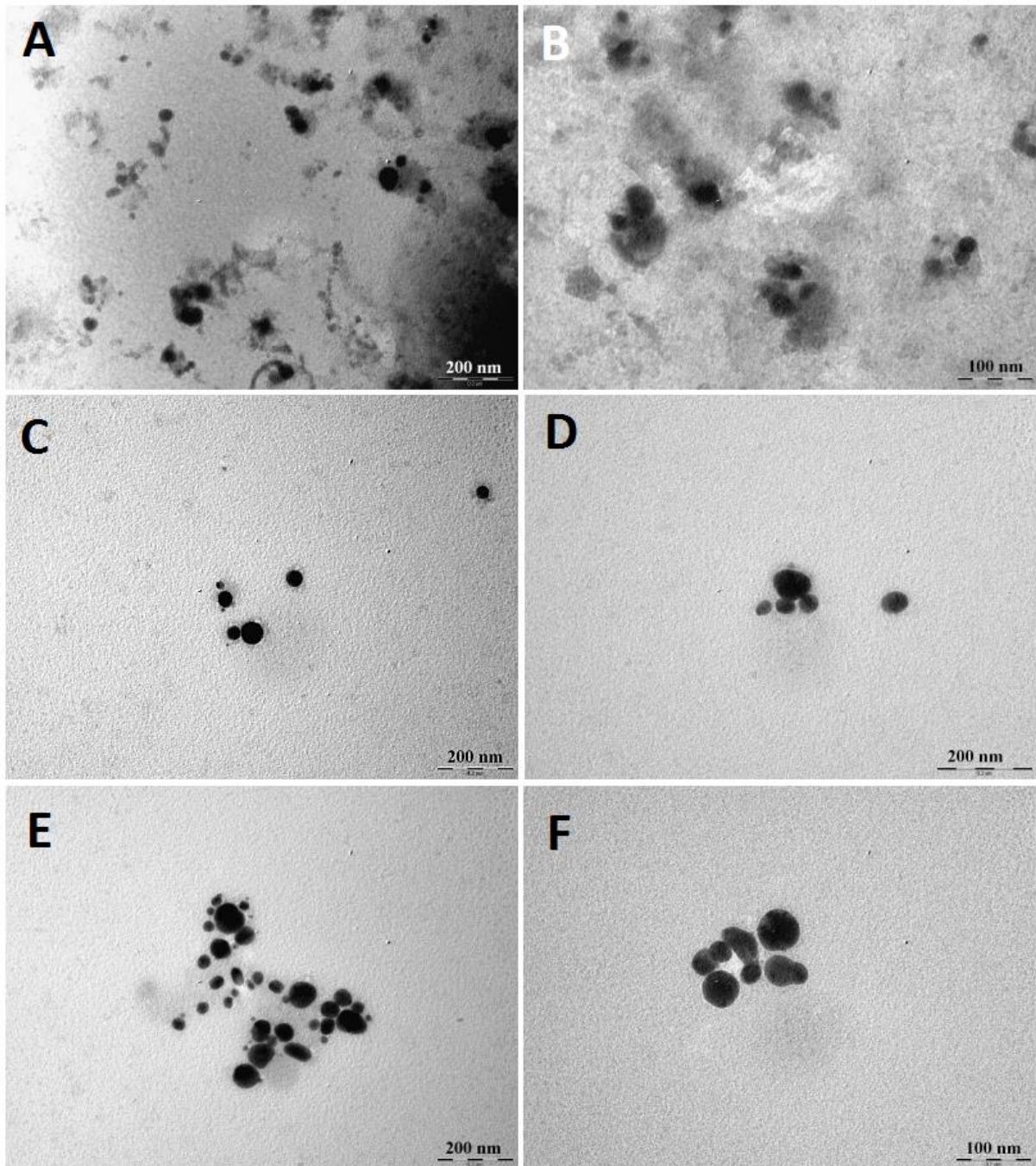
Slika 49. TEM mikrografije nanočestica srebra promjera 60 nm (Ag60 LMNB) dispergiranih u filtriranoj prirodnoj morskoj vodi saliniteta 15 (FSW 15) s dodatkom 10 \text{ mg mL}^{-1} Tweena 80. Svaka od slika (A-F) predstavlja mikrografiju istog uzorka. Koncentracija nanočestica bila je 5 \mu\text{g mL}^{-1} . Nanočestice su odstajale u mediju 48 sati, a eksperiment i snimanje izvršeni su pri sobnoj temperaturi.
