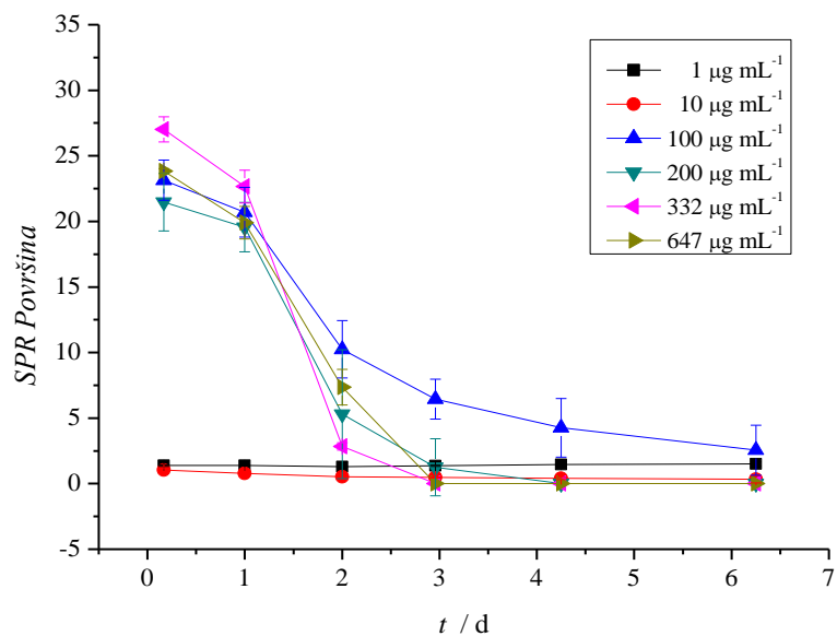
Slika 36. Promjene SPR površine pika nanočestica srebra promjera 60 nm (Ag60 NC, masene koncentracije 5 µg mL -1 ) kojima je dodan supernatant hemolimfe dagnje M. galloprovincialis različitog sadržaja proteina (1 – 647 µg mL -1 ) u umjetnoj morskoj vodi saliniteta 15 tijekom 6 dana pri sobnoj temperaturi.
