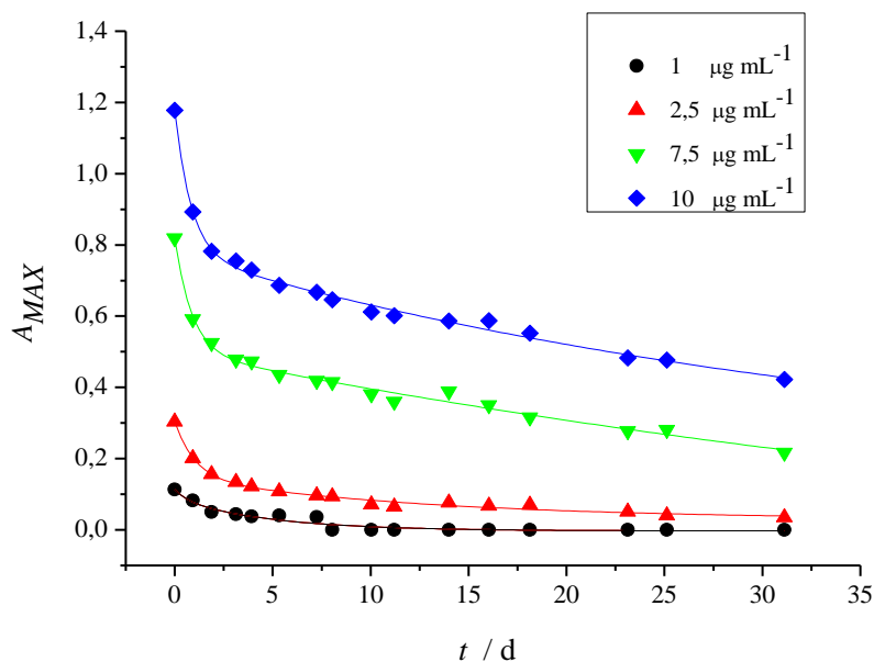
Slika 24. Vrijednosti apsorpcijskog maksimuma, A_{MAX} , za različite koncentracije ( 1 - 10 \mu\text{g mL}^{-1} ) nanočestica srebra promjera 40 nm (Ag40) s dodatkom BSA ( 100 \mu\text{M} ) u umjetnoj morskoj vodi saliniteta 38. Eksperiment i mjerenja provedeni su pri sobnoj temperaturi.
