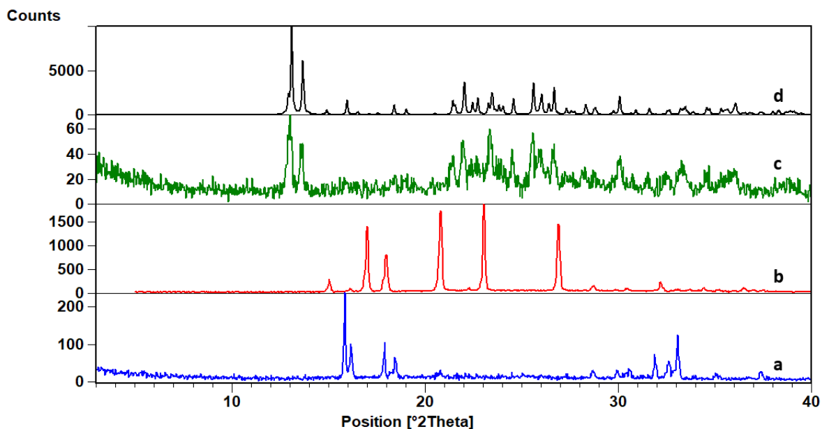
Slika D35. Difraktogrami: a) CoCl_2 \cdot 6H_2O , b) bpy, c) produkta dobivenog mljevenjem reakcijske smjese CoCl_2 \cdot 6H_2O , bpy i ipfb u stehiometrijskom omjeru 1:2:2, d) difraktogram izračunat iz podataka o kristalnoj i molekularnoj strukturi dobivenih difrakcijom u jediničnom kristalu (2)(ipfb)_2
