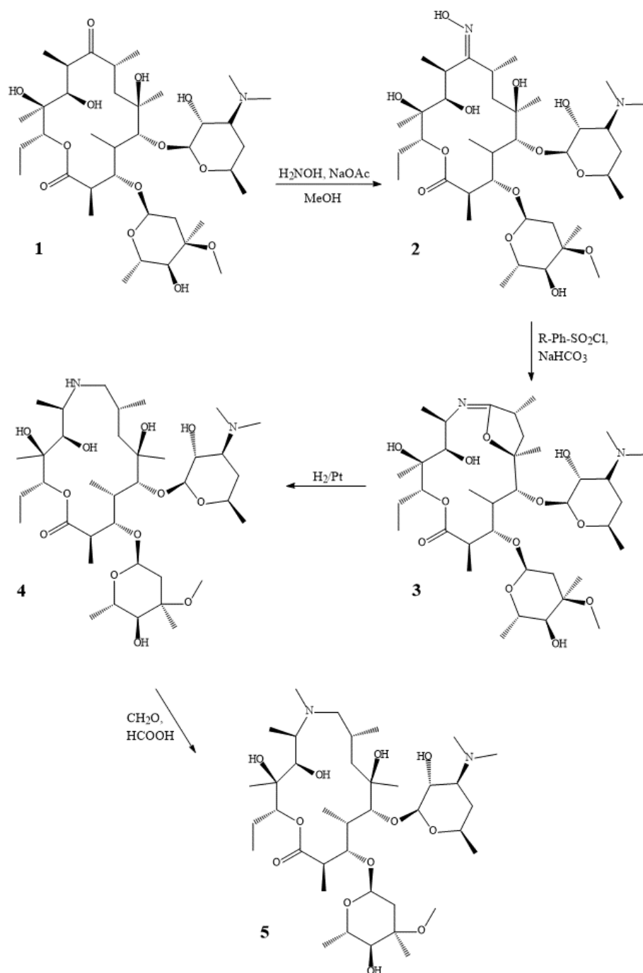
Shema 1. Sinteza azitromicina (1 – eritromicin A, 2 – eritromicin-9(E)-oksim, 3 – 6,9-iminoeter, 4 – 9-deokso-9dihidro-9a-aza-9a-homoeritromicin A, 5 – azitromicin).
